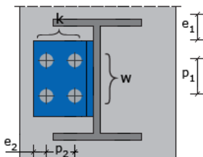
Mimośrodność działania sił
