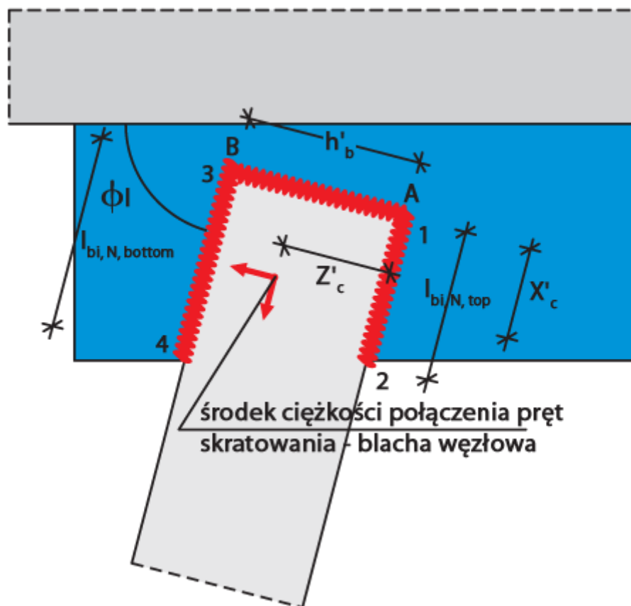
Punkty istotne układu spoin
