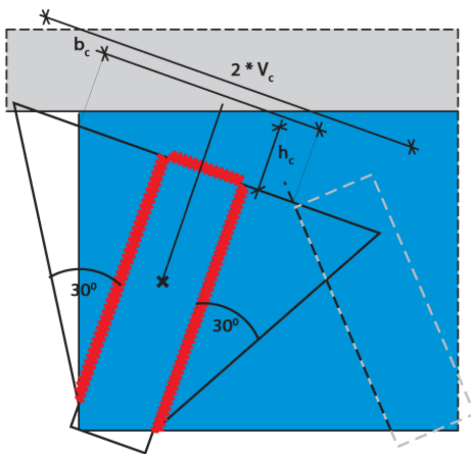
Rysunek schematyczny ogólny parametrów zasięgu przekroju miarodajnego
