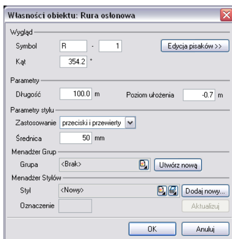
Rys 11. Okno własności rury osłonowej
