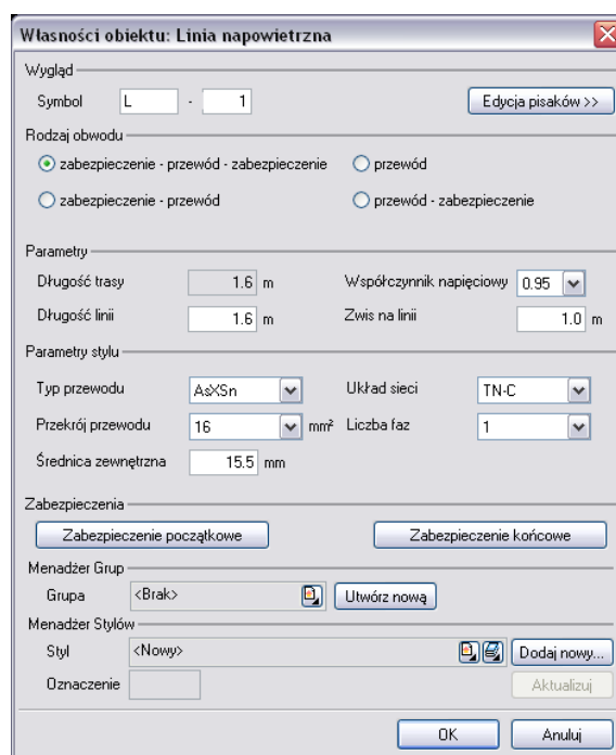
Rys 6. Okno własności linii napowietrznej
