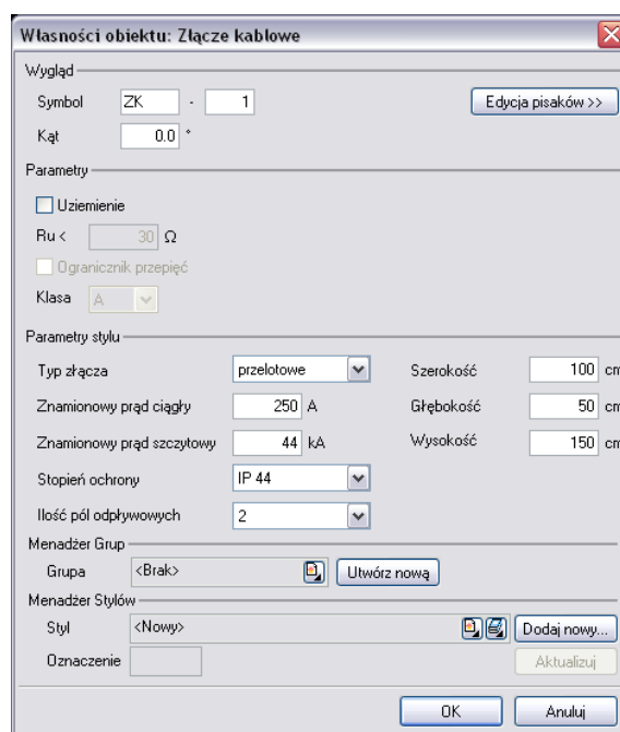
Rys 7. Okno własności złącza kablowego
