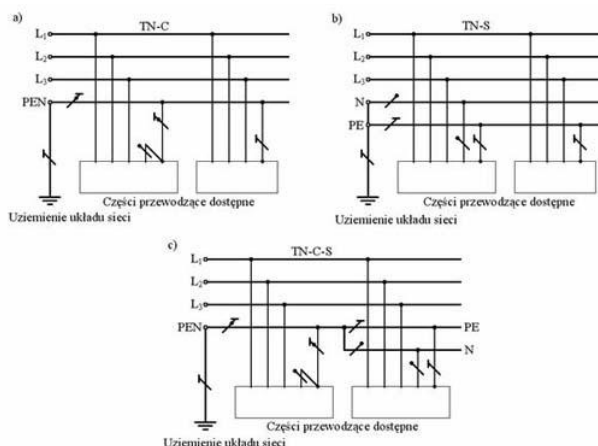
Rys 4. Schemat ideowy podukładów a) TN-C, b) TN-S i układ c) TN-C-S:
