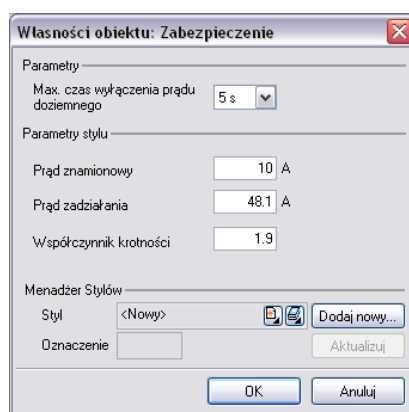
Rys 5. Okno własności zabezpieczenia
