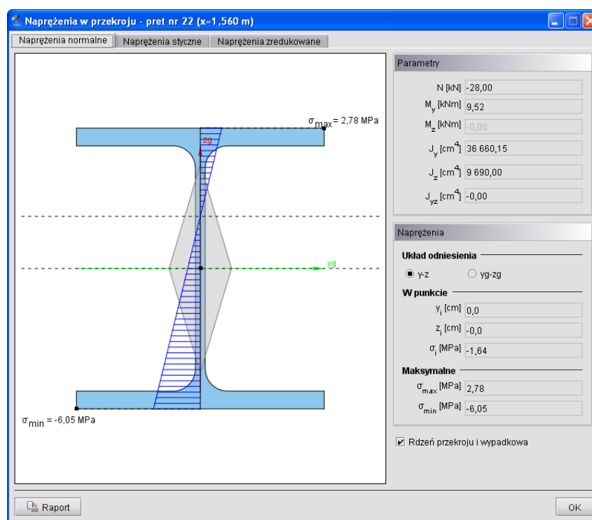
Rys. 3.45 Naprężenia normalne w przekroju
