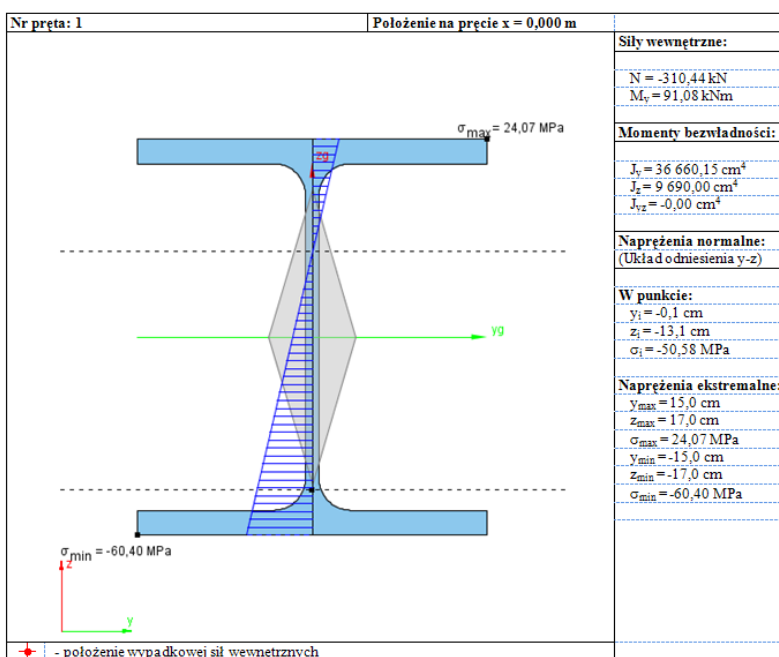
Rys. 3.46 Przykładowy raport dla naprężeń normalnych
