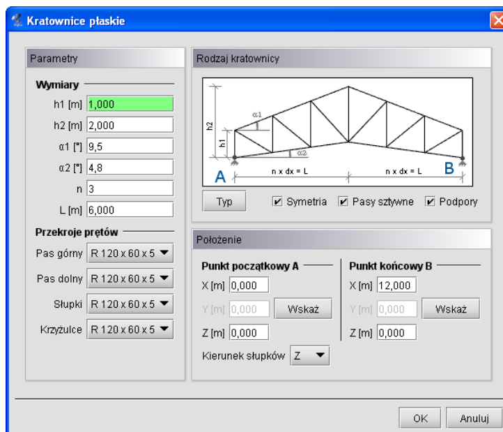
Rys. 3.30 Generator kratownic płaskich
