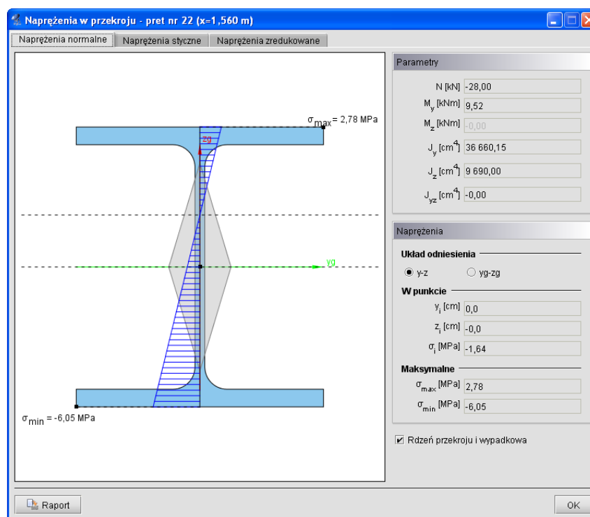
Rys. 3.44 Napężenia w przekroju
