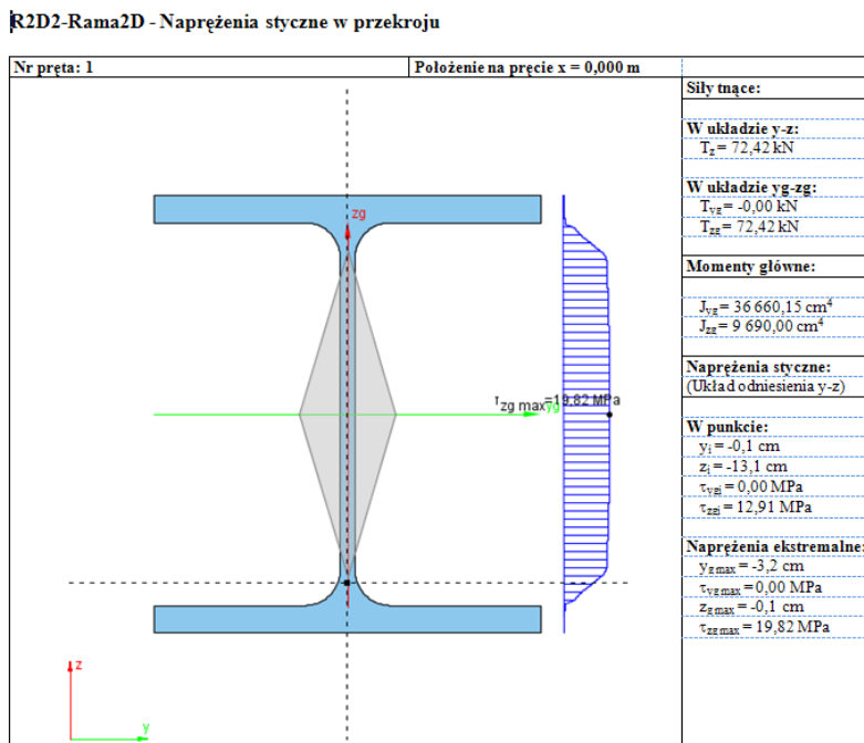
Rys. 3.48 Przykładowy raport z naprężeń stycznych w przekroju
