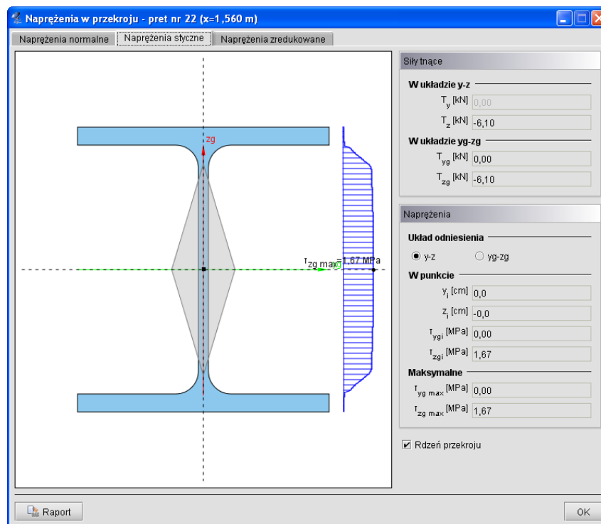
Rys. 3.47 Napężenia styczne w przekroju
