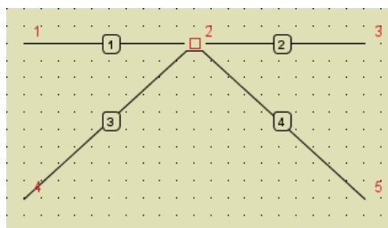
Pręty nr 3 i 4 zeszywnione
