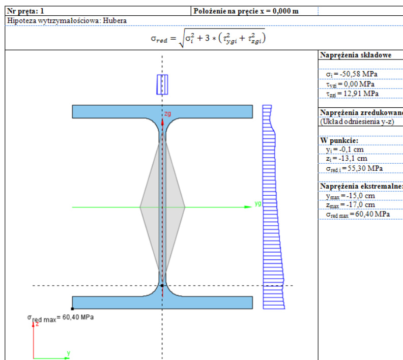
Rys. 3.50 Przykładowy raport z naprężeń zredukowanych w przekroju
