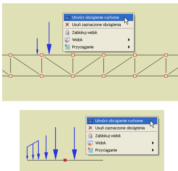
Rys. 7.10 Przykłady „zespołu pojazdu” z których można utworzyć obciążenie ruchome
