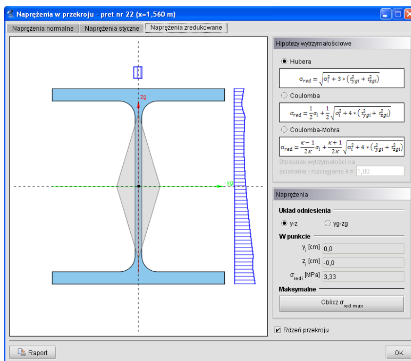
Rys. 3.49 Naprężenia zredukowane w przekroju
