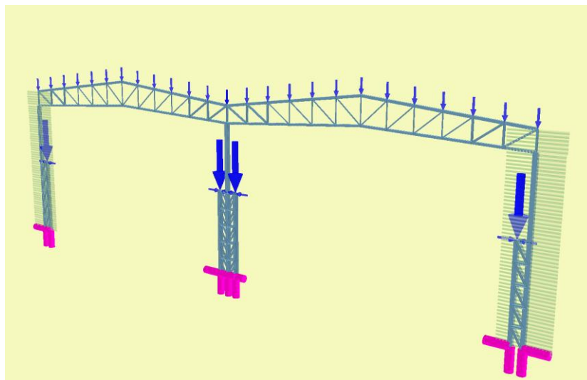
Rys. 13.5 Hala dwunawowa
