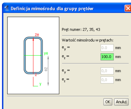
Rys. 9.4 Definicja mimośrodu dla grupy prętów
