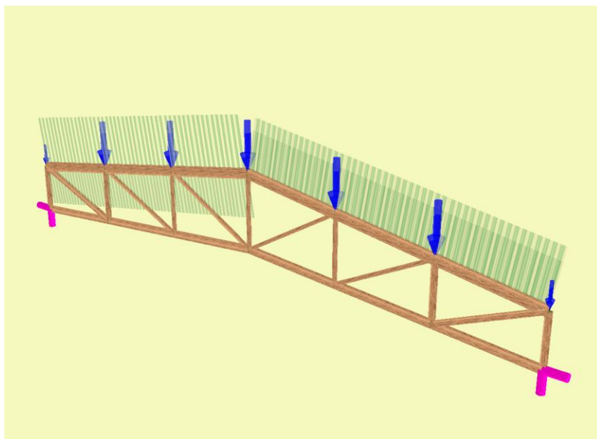
Rys. 13.1 Kratownica drewniana
