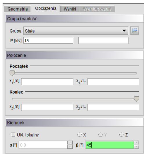
Rys. 7.8 Siły skupione węzłowe
