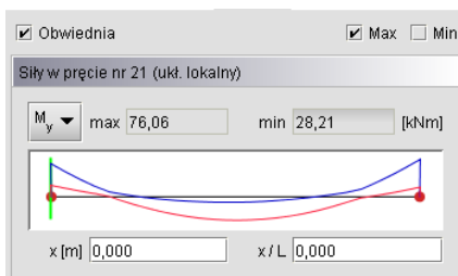
Rys. 11.6 Wykresy obwiedni dla pojedynczego przęta
