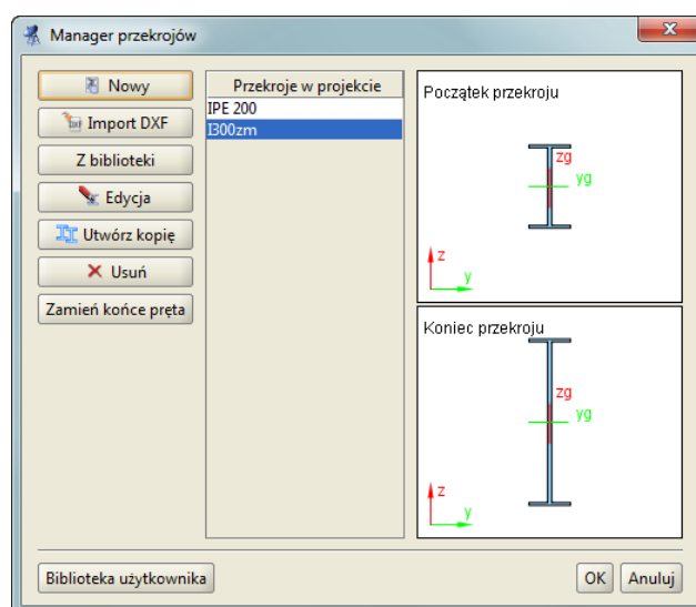
Rys. 4.12 Widok przekroju zmiennego w Managerze przekrojów
