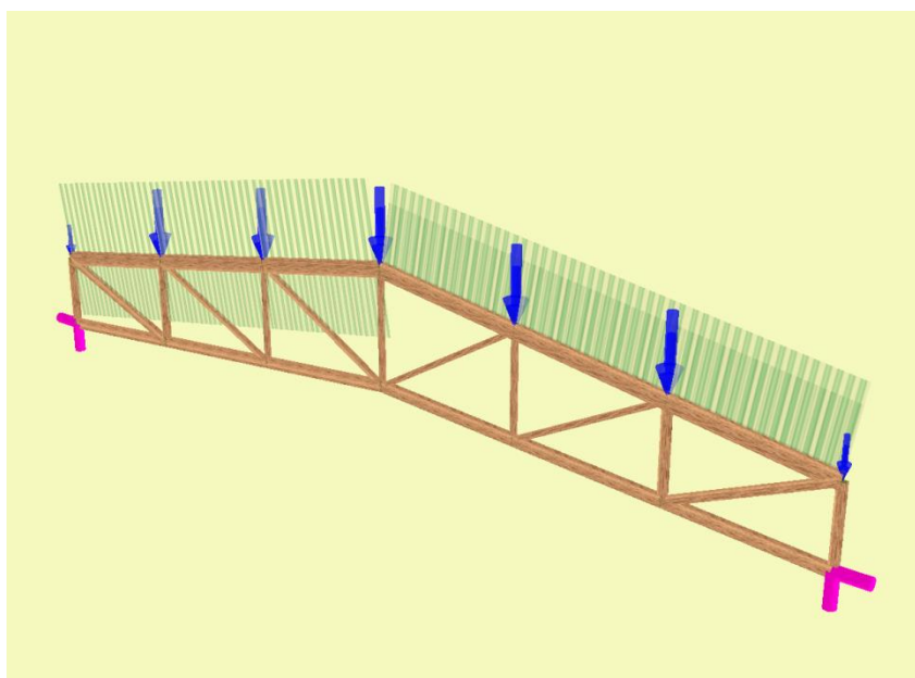
Rys. 13.1 Kratownica drewniana
