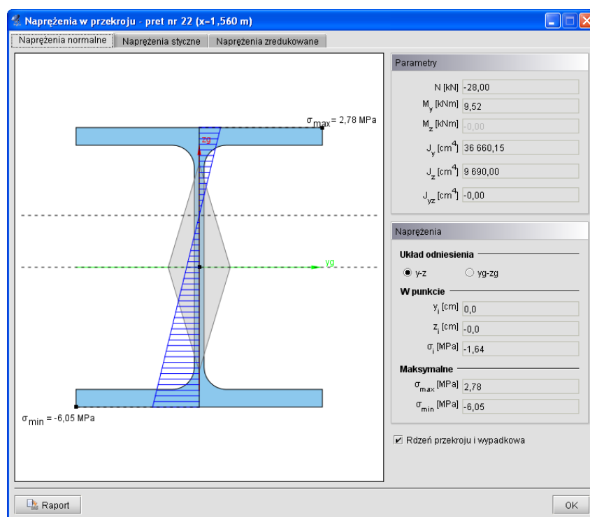
Rys. 3.59 Napężenia normalne w przekroju
