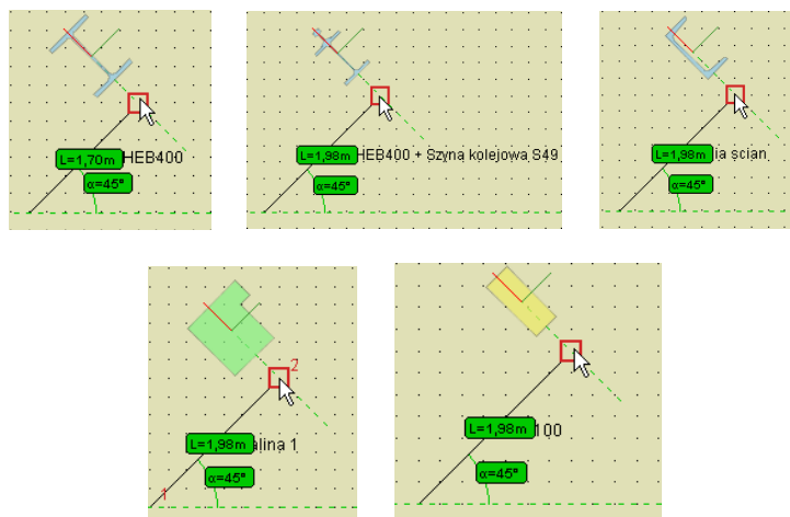
Rys. 3.36 Przykłady podglądu 2D przy wprowadzaniu elementu
