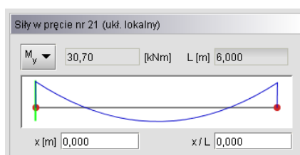
Rys. 11.4 Wykresy sił dla pojedynczego przęta
