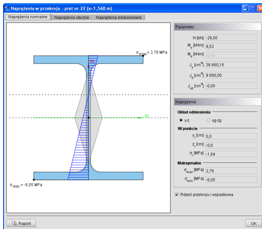
Rys. 3.58 Naprężenia w przekroju
