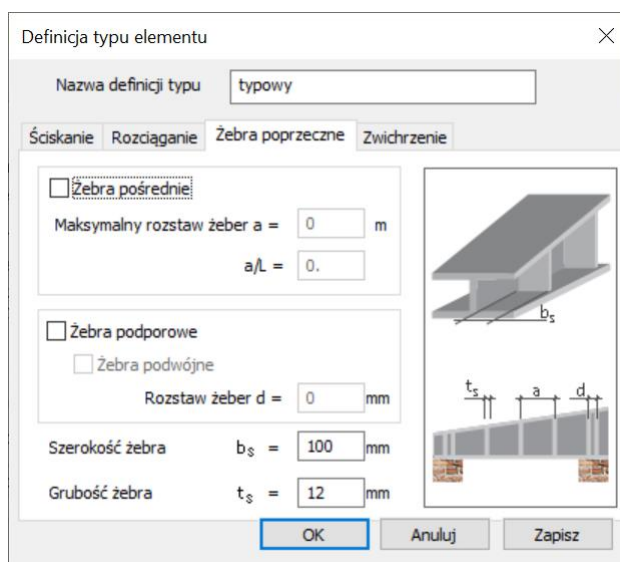
Rys. 2.7 Zakładka Żebra poprzeczne
