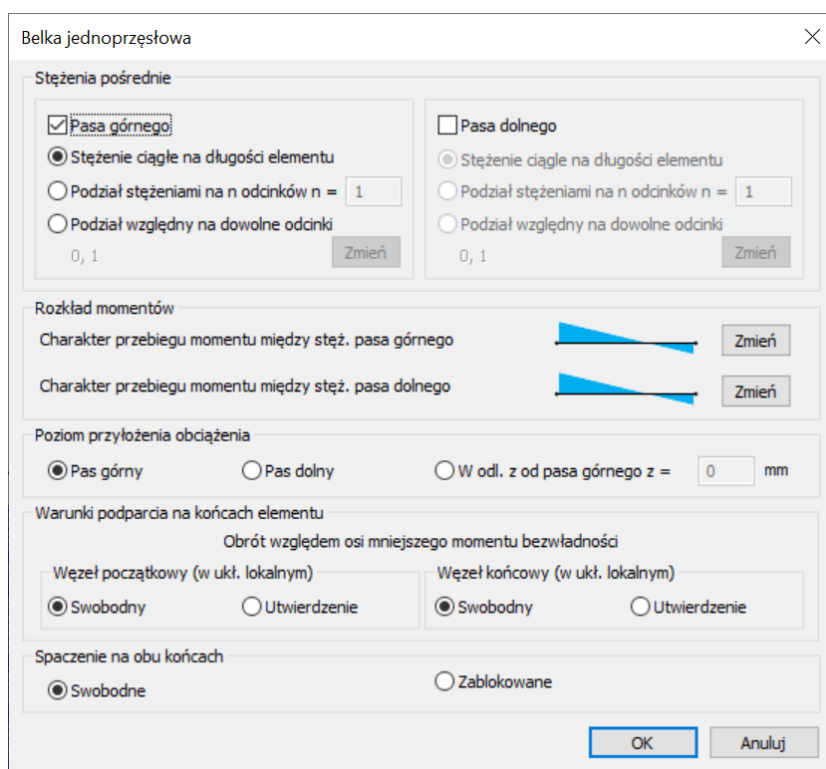
Rys. 2.9 Parametry belki
