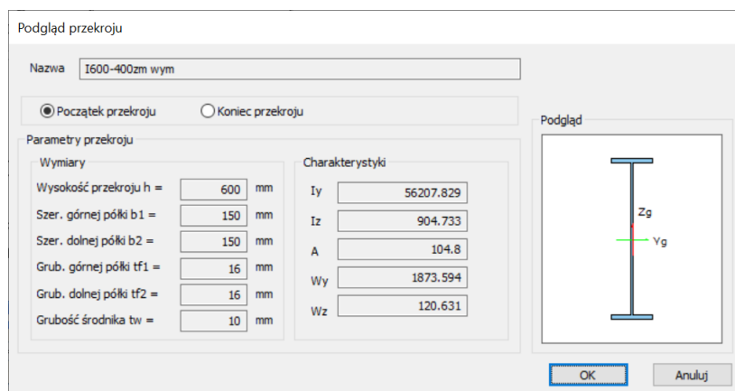
Rys. 2.2 Okno Podgląd przekroju
