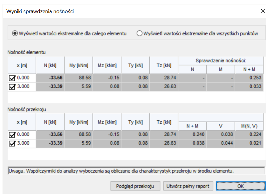
Rys. 2.13 Okno sprawdzania nośności
