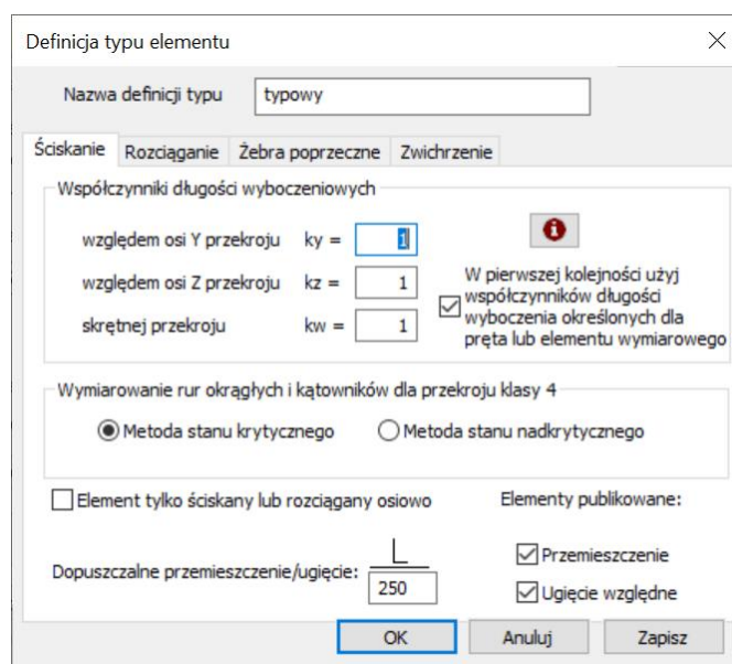
Rys. 2.5 Zakładka Ściskanie
