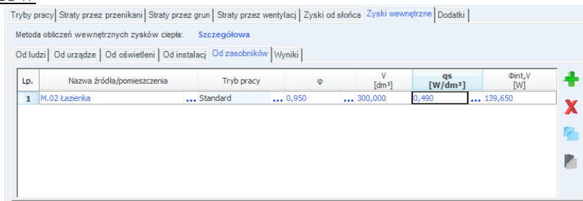
Rys 284. Zakładka wewnętrznych zysków ciepła metoda szczegółowa zyski od zasobników
