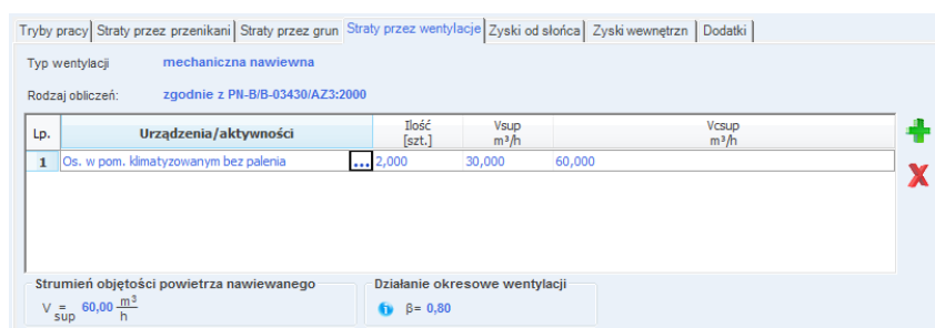
Rys 189. Zakładka straty na wentylację dla normy PN EN 13790:2008 wentylacja mech. nawiewna, wg normy PN-B/B-03430/AZ3:2000
