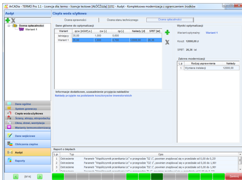
Rys 374. Zakładka oceny opłacalności ciepłej wody użytkowej.
