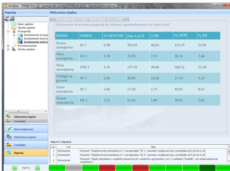
Rys 294. Raport zestawienie przegród w strefach ciepłych
