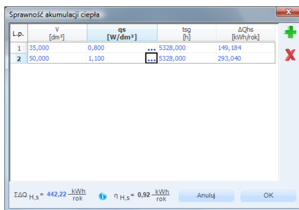
Rys 327. Okno umożliwiające obliczanie sprawności akumulacji
