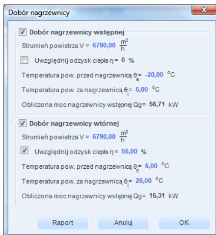
Rys 77. Okno doboru nagrzewnic
