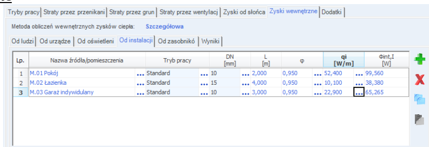
Rys 282. Zakładka wewnętrznych zysków ciepła metoda szczegółowa zyski od instalacji
