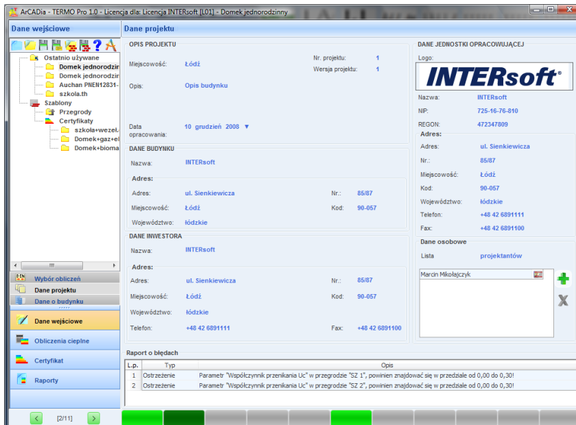
Rys 6. Okno dane projektu
