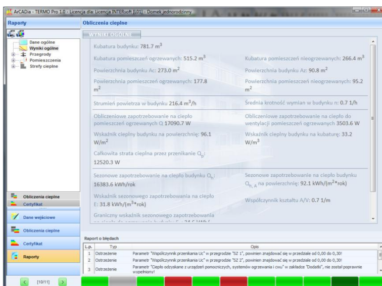
Rys 278. Raport wyniki ogólne
