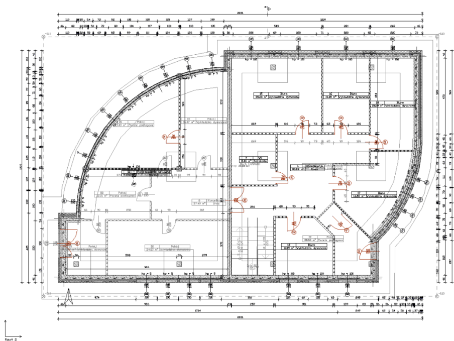
Rys. 29 Rzut parteru wraz z podglądem pozostałych kondygnacji projektu
