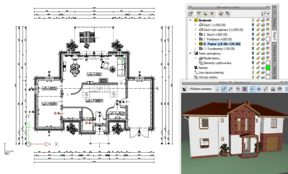
Rys. 43 Przykład z aktywnym widokiem: Rzut 1 i Widokiem 3D w trybie uproszczonym
