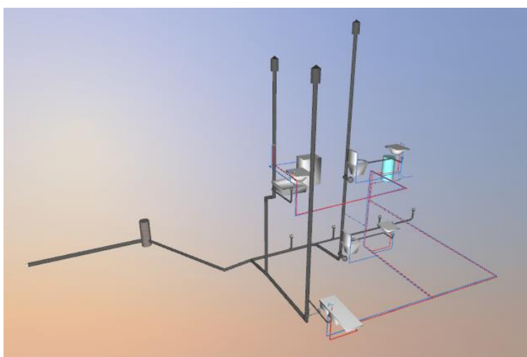
Rys. 69 Instalacja wod.-kan. w widoku z powierzchniami zdefiniowanymi w elementach
