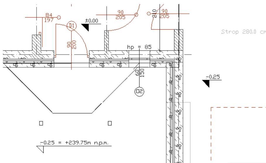
Rys. 111 Przykład projektu z opisem wysokości
