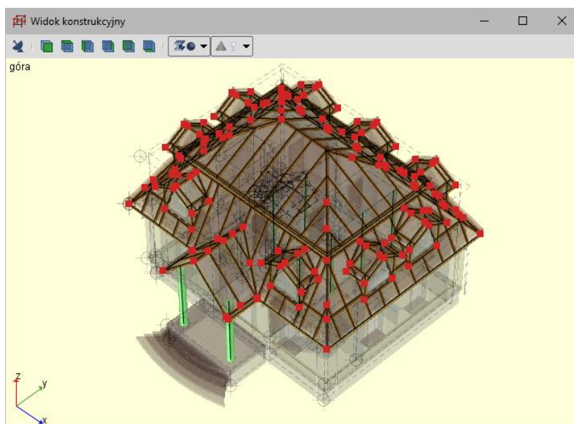
Rys. 220 Przykładowy projekt w widoku konstrukcyjnym
