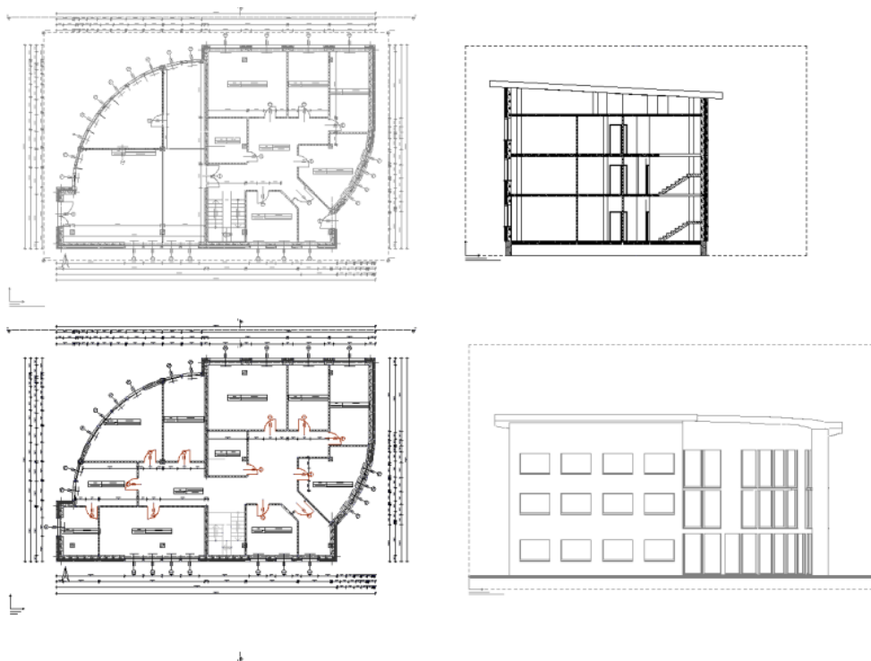
Rys. 31 Widoki. Na każdym widoku włączona jest tylko jedna kondygnacja.
