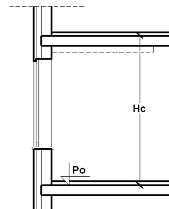
Rys. 100 Schemat danych kondygnacji, gdzie H_c jest wysokością całkowitą kondygnacji, a P_o wysokością bazową (poziomym odniesieniem)
