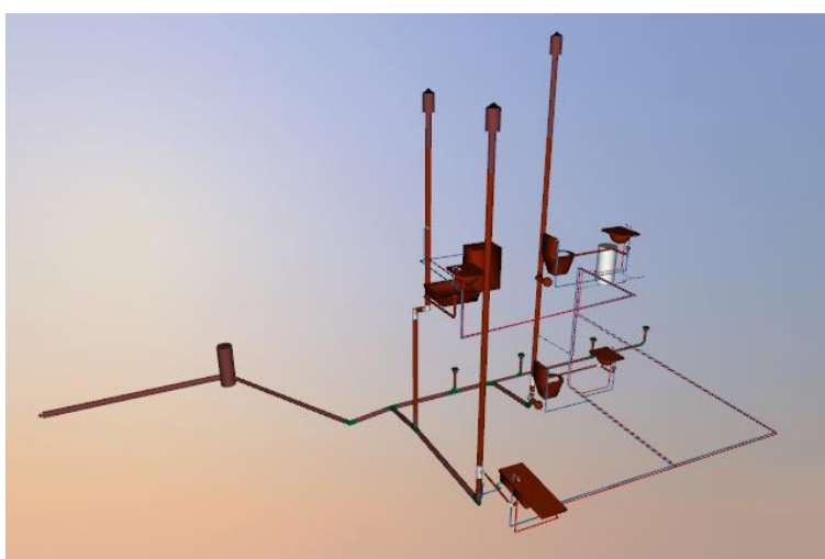
Rys. 70 Instalacja wod.-kan. w widoku koloru warstw z Menadżera projektu
