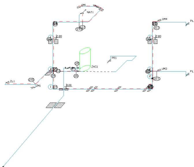
Rys. 37 Przykład aksonometrii instalacji wodociągowej w domku jednorodzinny
