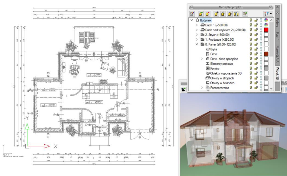
Rys. 49 Pokazanie przezroczystości dla elementów w starym silniku
