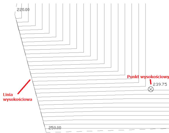
Rys. 115 Elementy terenu na rzucie
