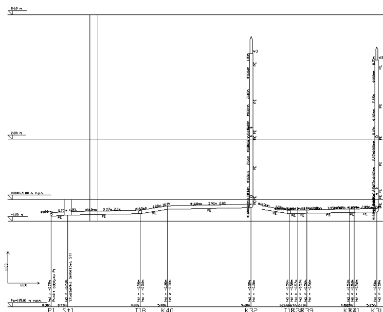
Rys. 38 Przykład profilu instalacji kanalizacyjnej
