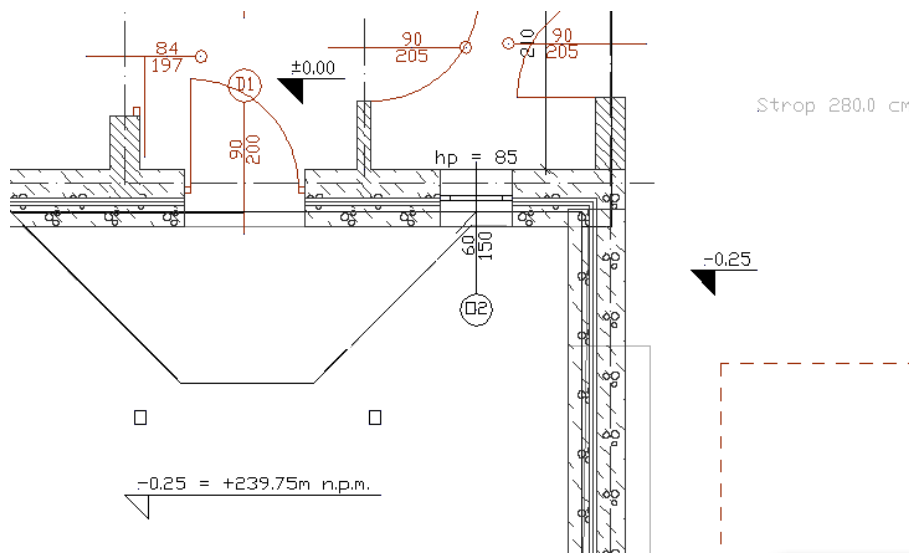
Rys. 84 Przykład projektu z opisem wysokości
