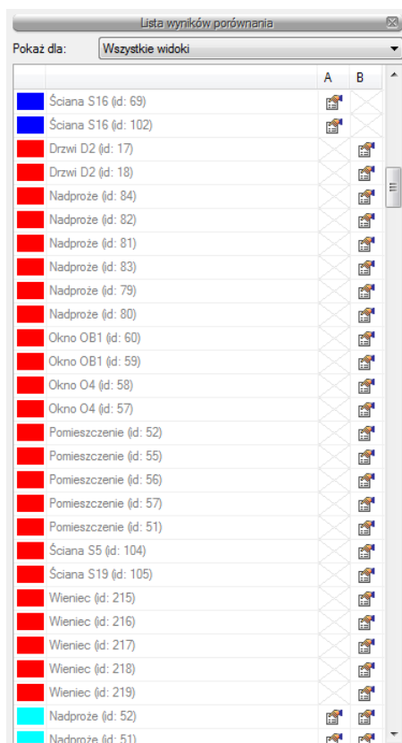
Rys. 59 Lista elementów nowych i zmienionych w porównywanych dokumentach
