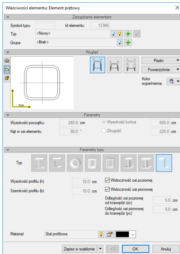
Rys. 184 Okno jednego z elementów rozbitego szkieletu zaimportowanej konstrukcji prętowej.
