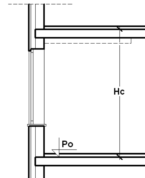
Rys. 73 Schemat danych kondygnacji, gdzie Hc jest wysokością całkowitą kondygnacji, a Po wysokością bazową (poziomem odniesienia)
