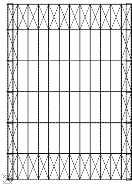
Rys. 183 Przykład zaimportowanego do programu szkieletu konstrukcji
