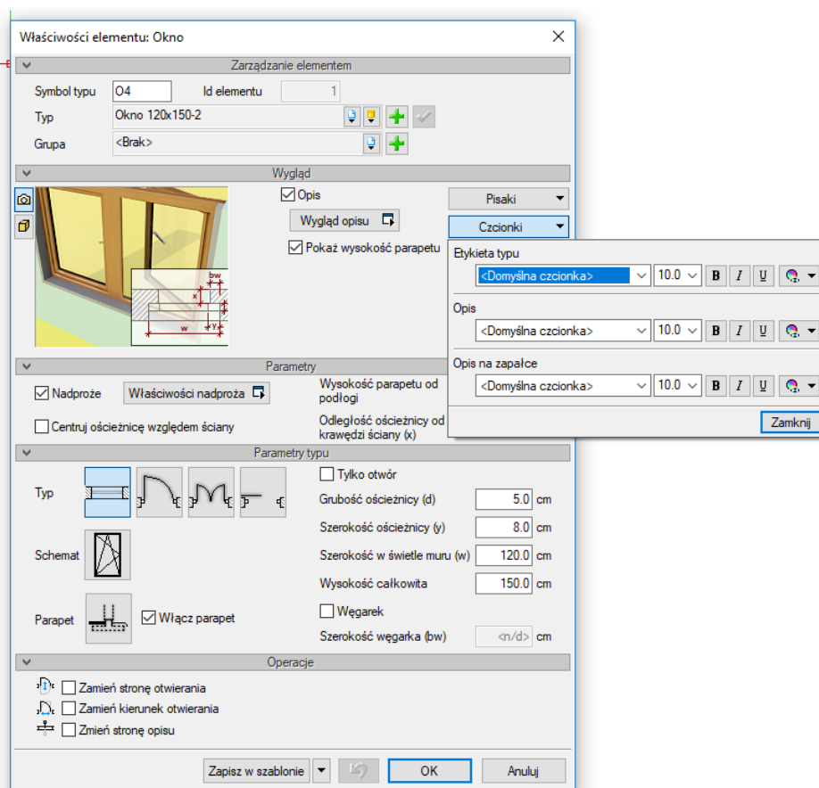
Rys. 131 Okno dialogowe właściwości okna z rozwiniętą listą dostępnych czcionek opisu
