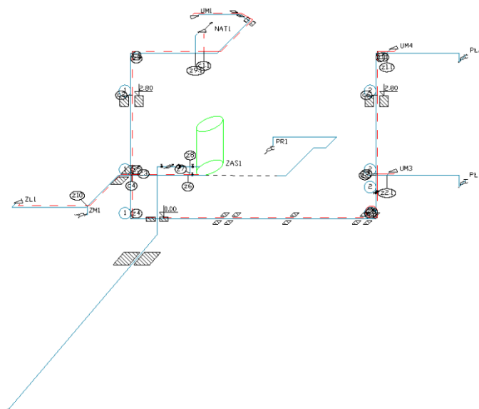
Rys. 32 Przykład aksonometrii instalacji wodociągowej w domku jednorodzinnym
