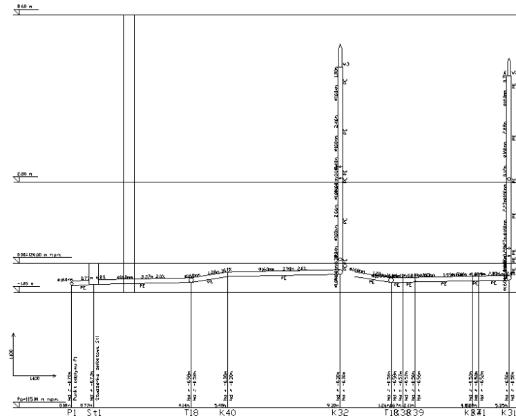
Rys. 33 Przykład profilu instalacji kanalizacyjnej
