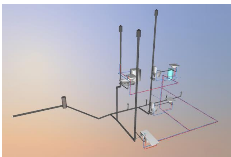
Rys. 46 Instalacja wod.-kan. w widoku z powierzchniami zdefiniowanymi w elementach
