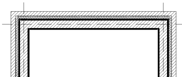
Rys. 129 Ściana z pisakiem Linia oddzielająca warstwę nośną ściany na 0,5 a Obrys przecięcia z płaszczyzną rzutu/przekroju na 0,18 a (jak pozostałe pisaki)
