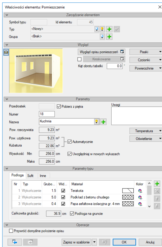
Rys. 79 Okno właściwości przykładowego pomieszczenia
