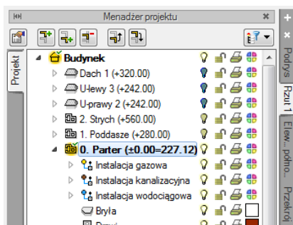
Rys. 74 Zaznaczenie kondygnacji z okna menadżera
