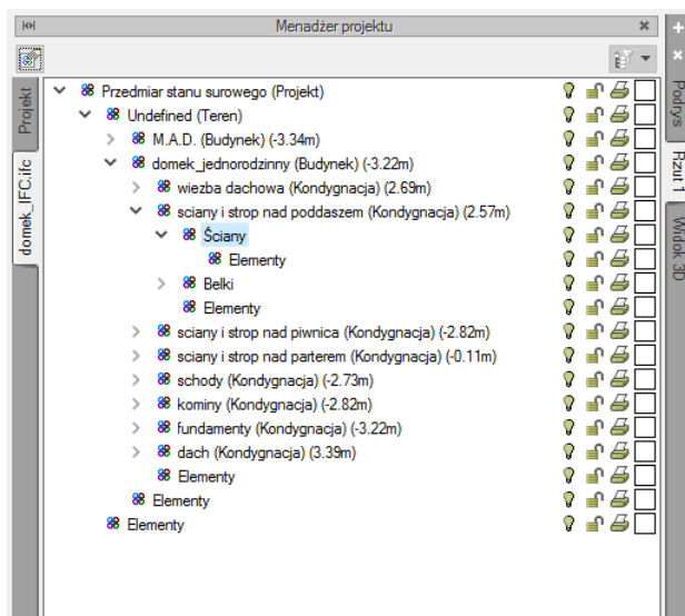
Rys. 173 Okno Menadżer projektu, zakładki modelu IFC po rozwinięciu i zaznaczeniu obiektów
