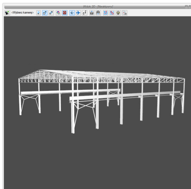
Rys. 183 Przykład zaimportowanego do programu szkieletu konstrukcji
