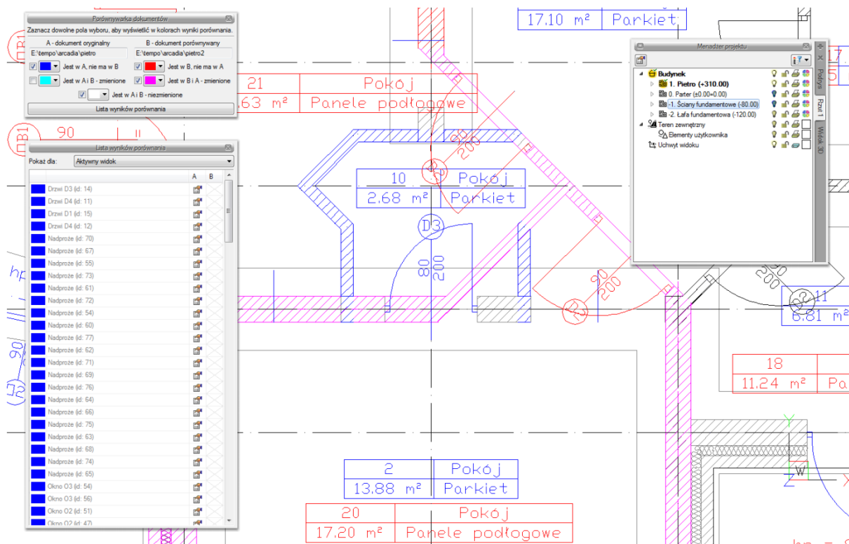
Rys. 61 Porównywane dokumenty z widocznymi zmienionymi elementami z dokumentu 2
