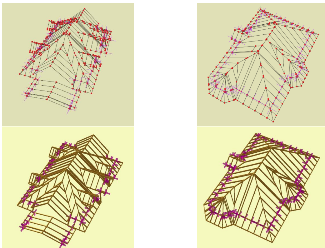
Rys. 2.42 Przykłady projektów dachów z systemu ArCADia z automatycznie wygenerowanym układem konstrukcji połączeń w modelu siatkowym i widoku 3D
