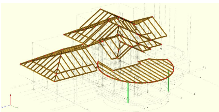
Rys. 2.13 Widok wyłączonego modelu z ArCADii z renderowanym widokiem prętów i włączonym wyświetlaniem podrysów
