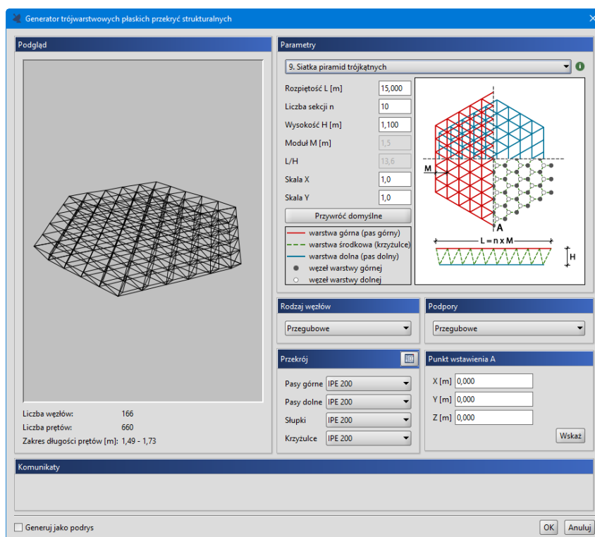
Rys. I.23 Okno Generatora trójwarstwowych płaskich przekryć strukturalnych
