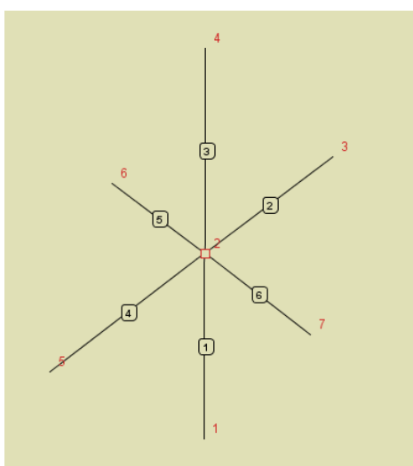
Rys. 3.89 Trzy grupy prętów zeszywnionych połączone między sobą przegubami
