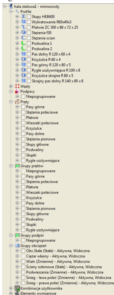
Rys. 2.15 „Drzewo projektu”
