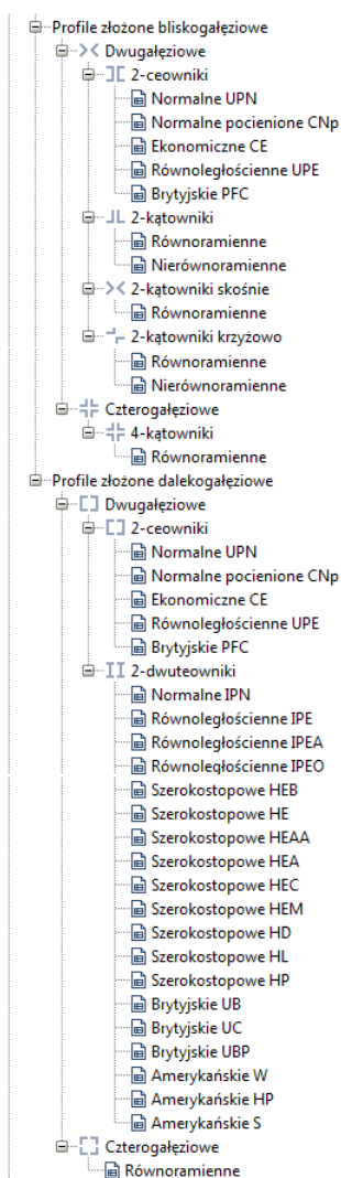
Rys. 4.16 Profile wielogąłęziowe – wymiarowane
