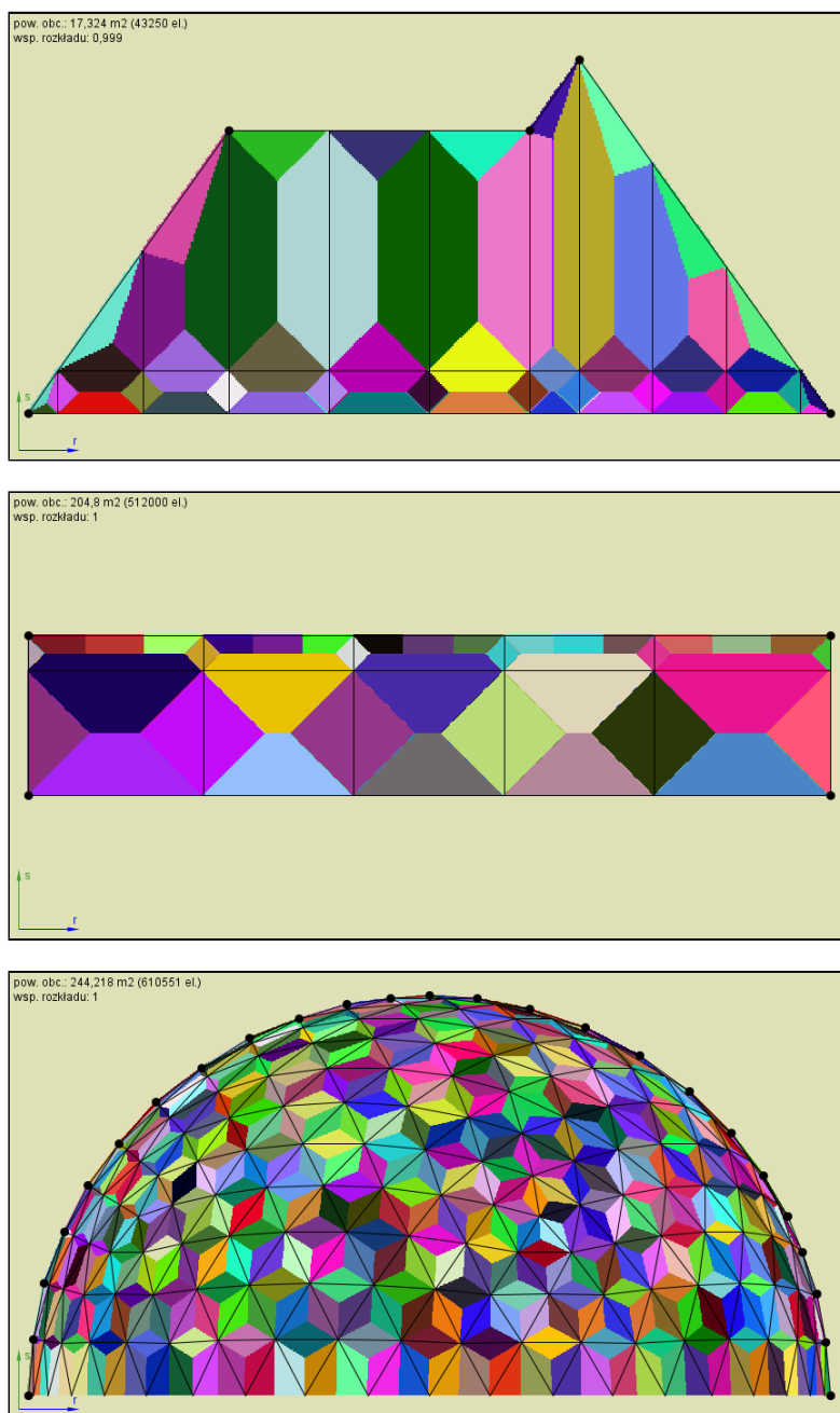
Rys. 7.44 Przykłady podglądu rozkładu obciążenia powierzchniowego
