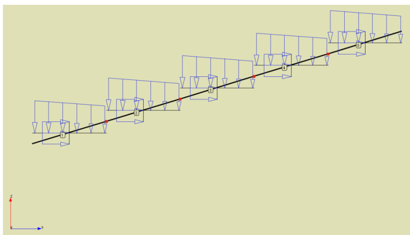
Rys. 7.14 Reprezentacja graficzna obciążeń zadawanych na rzut prętów
