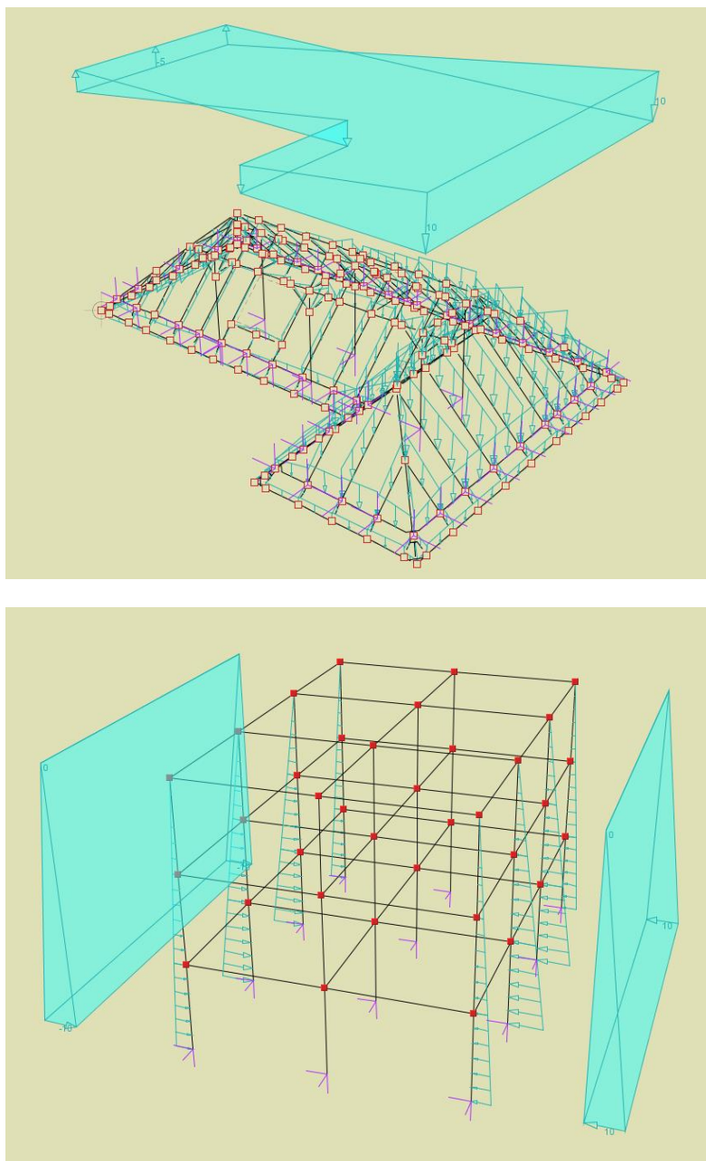
Rys. 7.41 Przykłady zdefiniowanego obciążenia powierzchniowego trapezowego
