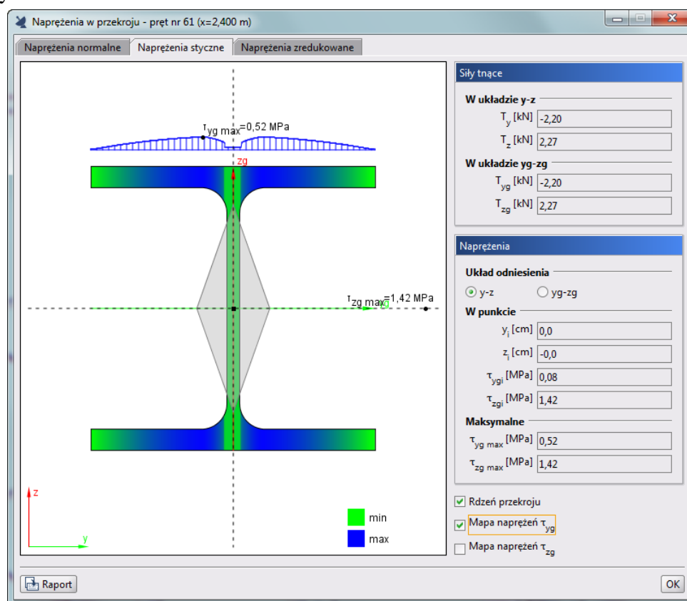
Rys. 3.73 Naprężenia styczne w przekroju
