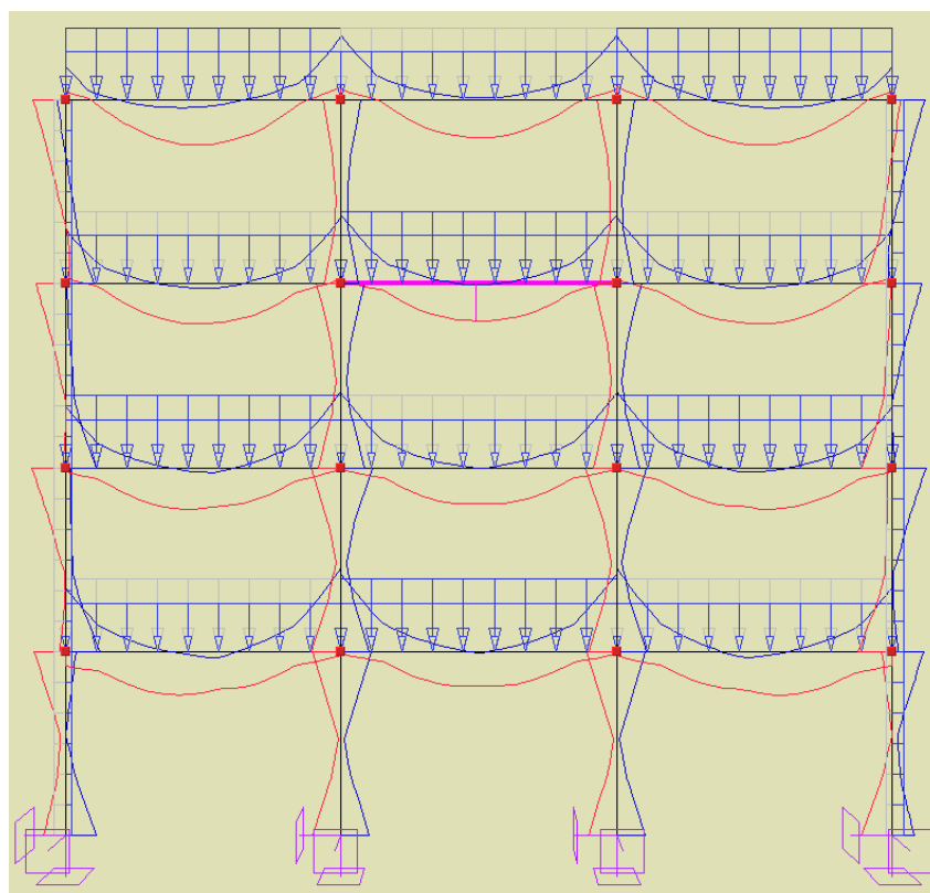
Rys. 3.12 Schemat obciążeń budujący ekstremum gnącego momentu przęsłowego w zaznaczonym ryglu
