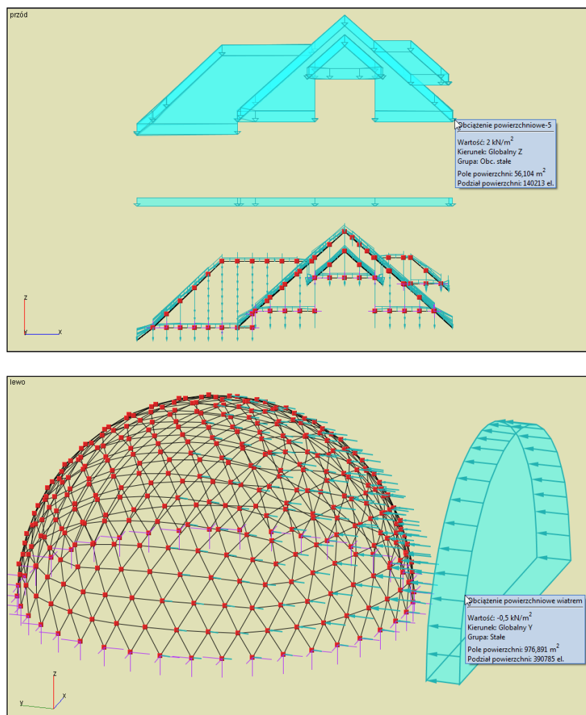
Rys. 7.48 Przykłady zadanych obciążeń powierzchniowych
