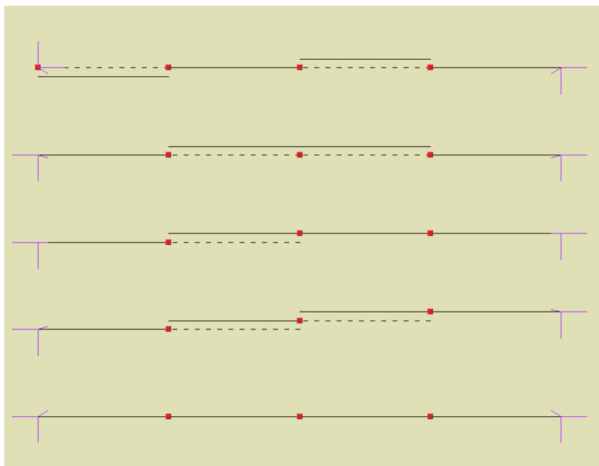
Rys. 7.21 Układy prętów z mimośrodami, na których można wprowadzić obciążenie ruchome
