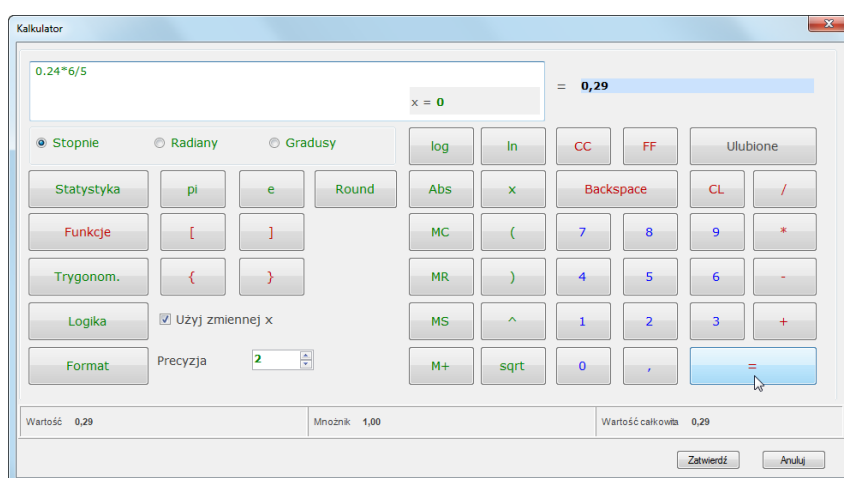
Rys. 7.56 Kalkulator matematyczny
