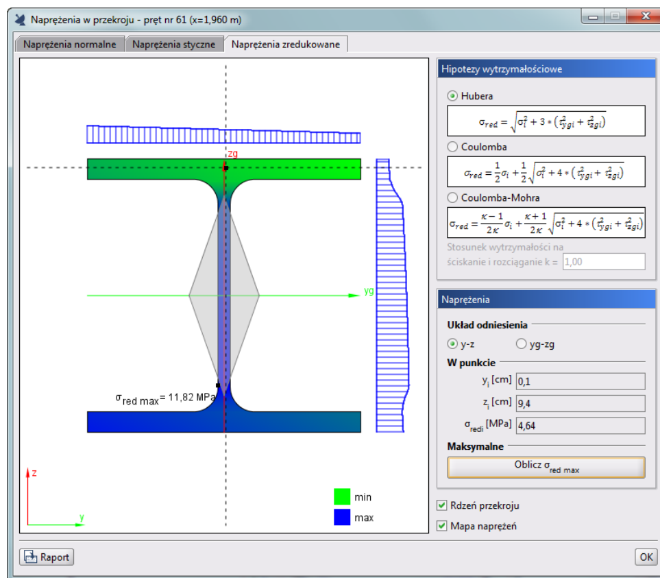
Rys. 3.64 Naprężenia zredukowane w przekroju
