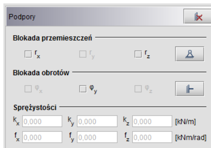
Rys. 6.3 Podpory
