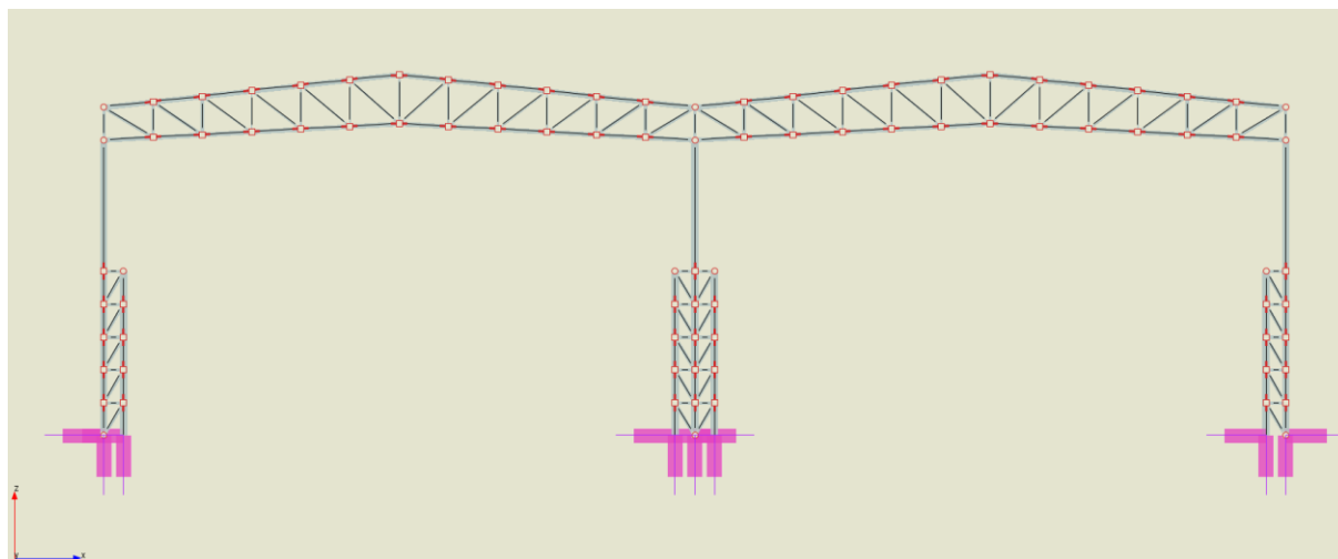
Rys. 2.4 Widok przezroczysty przekrojów prętów
