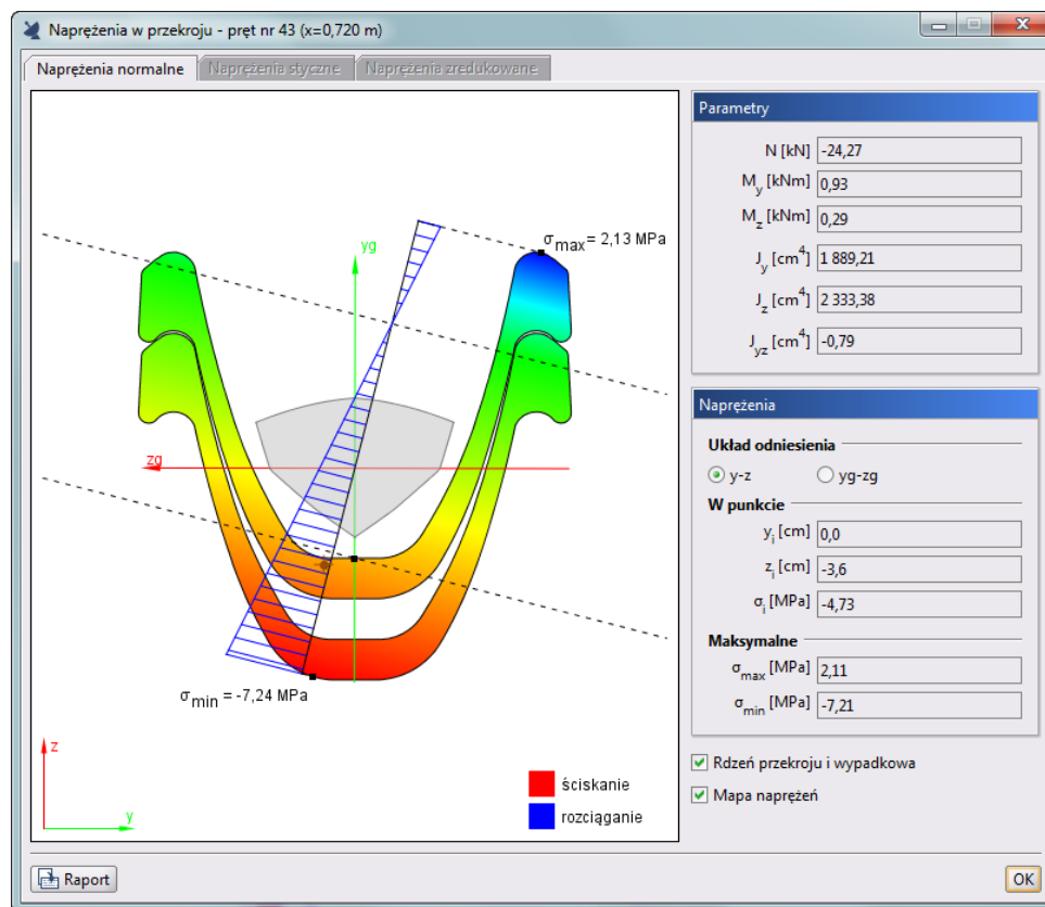
Rys. 3.60 Naprężenia normalne w przekroju
