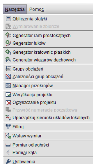
Rys. 3.39 Menu Narzędzia
