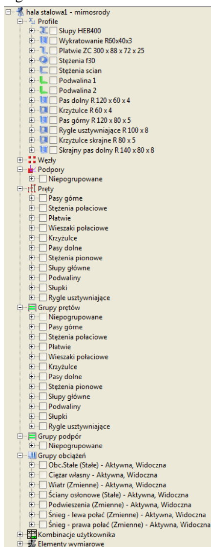
Rys. 2.7 Drzewo projektu
