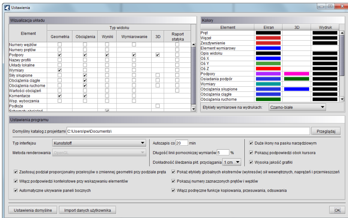
Rys. 3.71 Okno Ustawień
