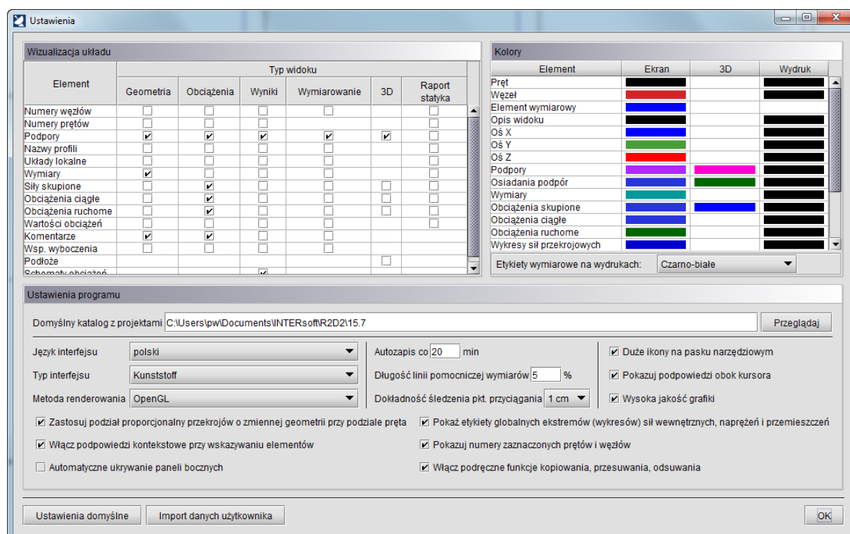
Rys. 3.70 Ustawienia programu
