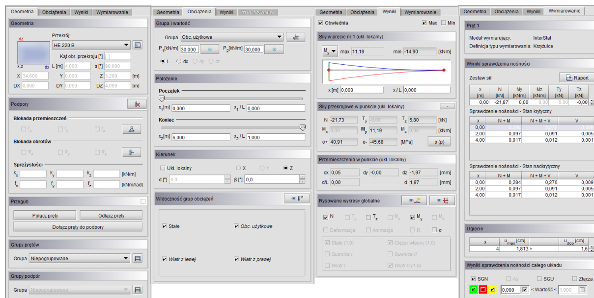
Rys. 2.6 Zakładki programu
