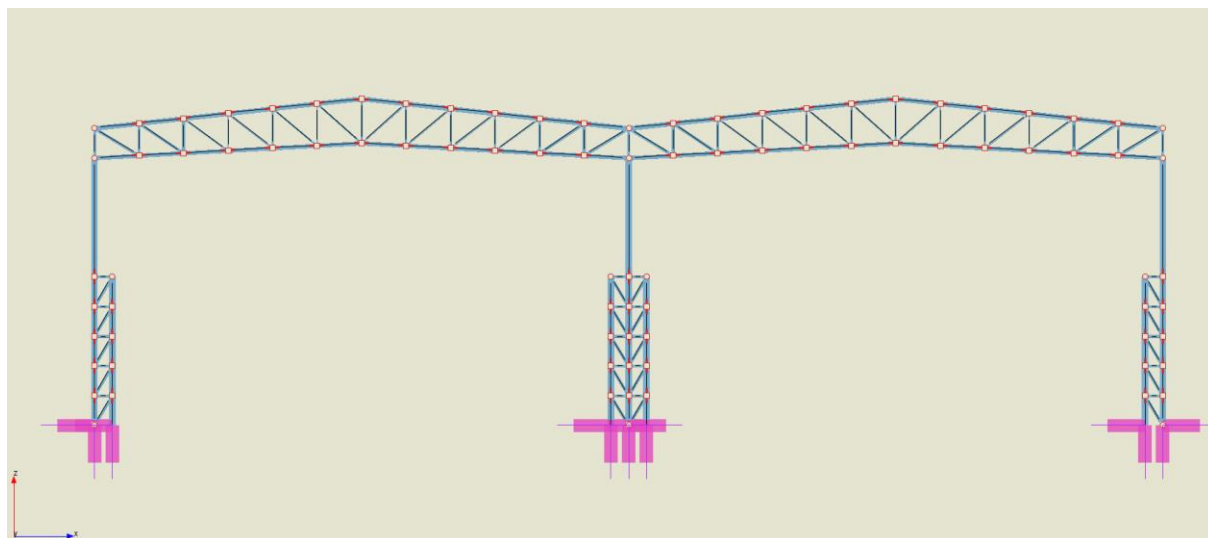
Rys. 2.3 Widok teksturowany przekrojów prętów
