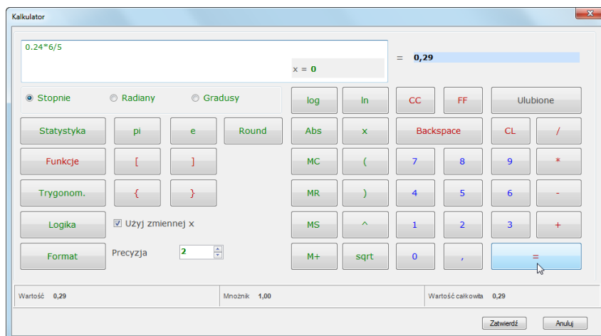
Rys. 7.40 Kalkulator matematyczny
