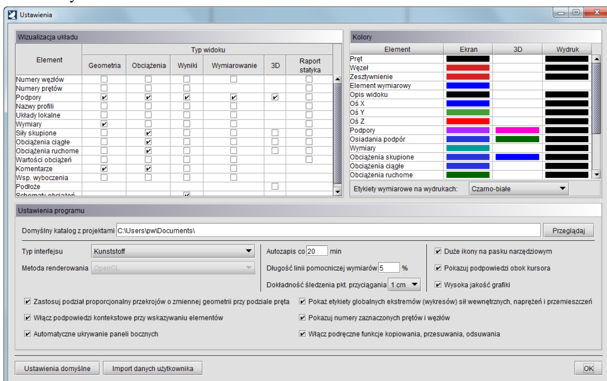
11.17 Okno Ustawień
