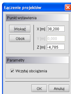
Rys. 2.12 Łączenie projektów
