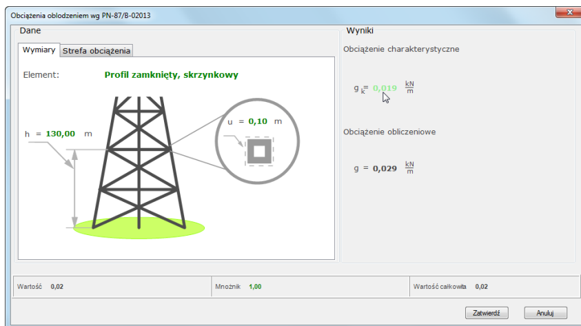
Rys. 7.39 Kalkulator obciążenia oblodzeniem wg normy PN
