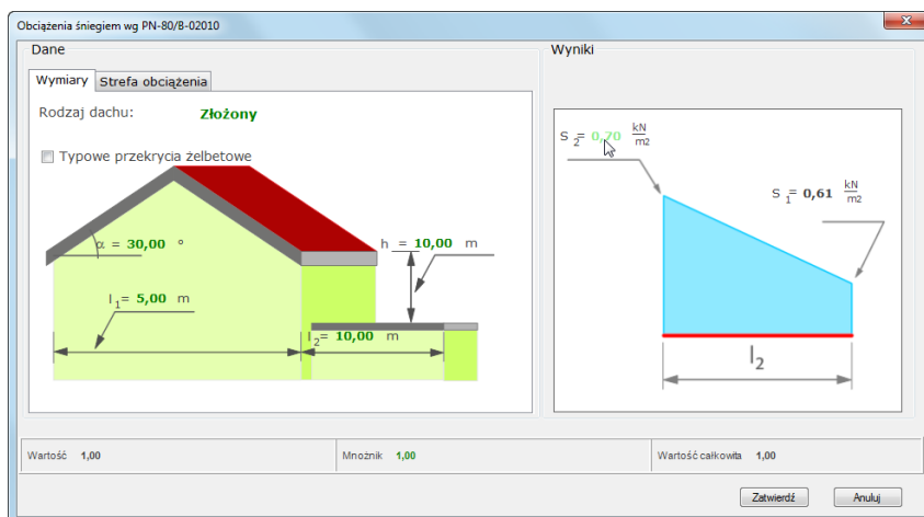
Rys. 7.37 Kalkulator obciążenia śniegiem wg normy PN
