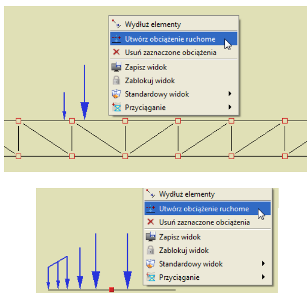
Rys. 7.15 Przykłady „zespołu pojazdu” z których można utworzyć obciążenie ruchome
