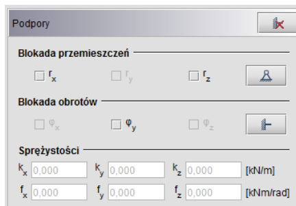
Rys. 6.3 Podpory
