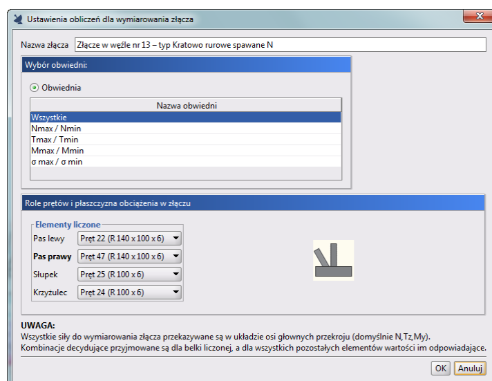
Rys. 14.44 Okno definicji złącza Kratowo rurowe spawanego typu N
