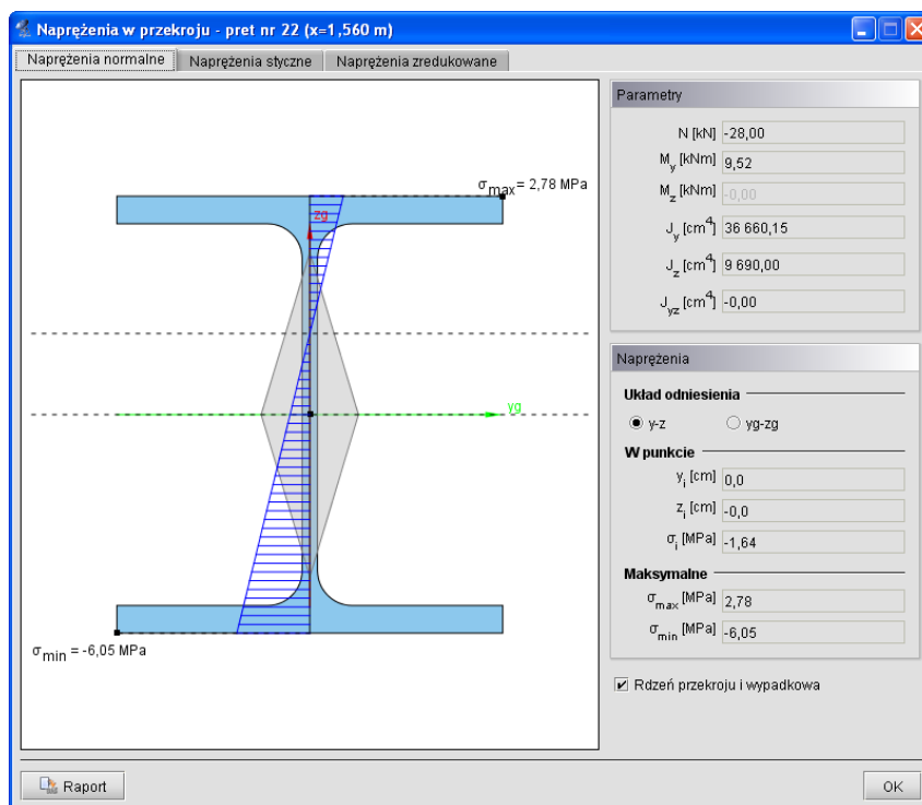
Rys. 3.59 Napężenia w przekroju
