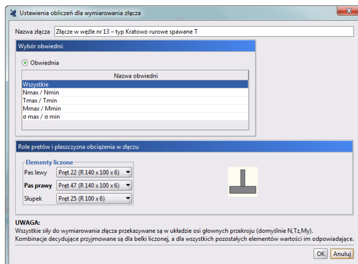
Rys. 14.45 Okno definicji złącza Kratowo rurowe spawanego typu T
