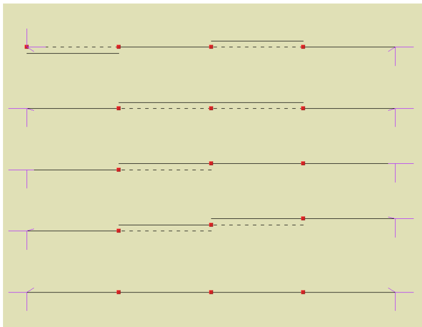
Rys. 7.16 Układy prętów z mimośrodami na których można wprowadzić obciążenie ruchome
