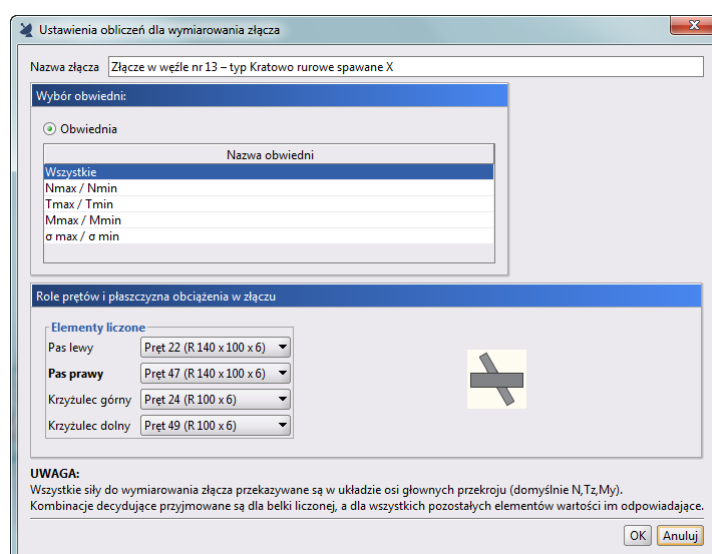
Rys. 14.46 Okno definicji złącza Kratowo rurowe spawanego typu X
