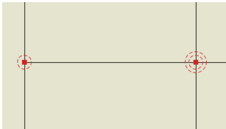
Rys. 14.48 Widok złączy (pojedynczego i podwójnego) zdefiniowanych w węzłach modelu statycznego
