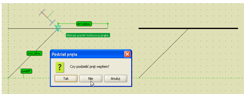
Rys. 3.75 Wprowadzany pręt niepołączony (luźny)
