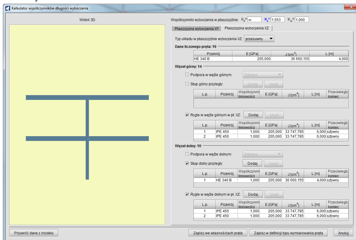
Rys. 3.78 Okno kalkulatora współczynników długości wyboczeńowych
