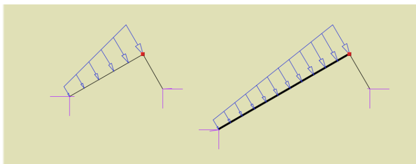
Rys. 3.56 Wydłużenie o podaną wartość pręta podpartego o końcu swobodnym
