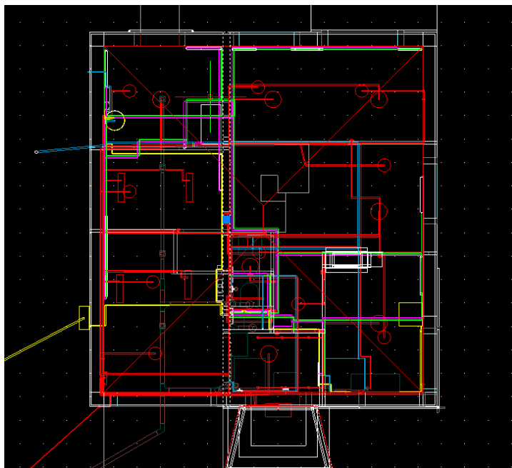
Rys. 254 Widok rzutu modelu IFC wprowadzonego z opcją Obwiednia obiektu
