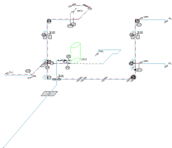
Rys. 62 Przykład aksonometrii instalacji wodociągowej w domku jednorodzinnym
