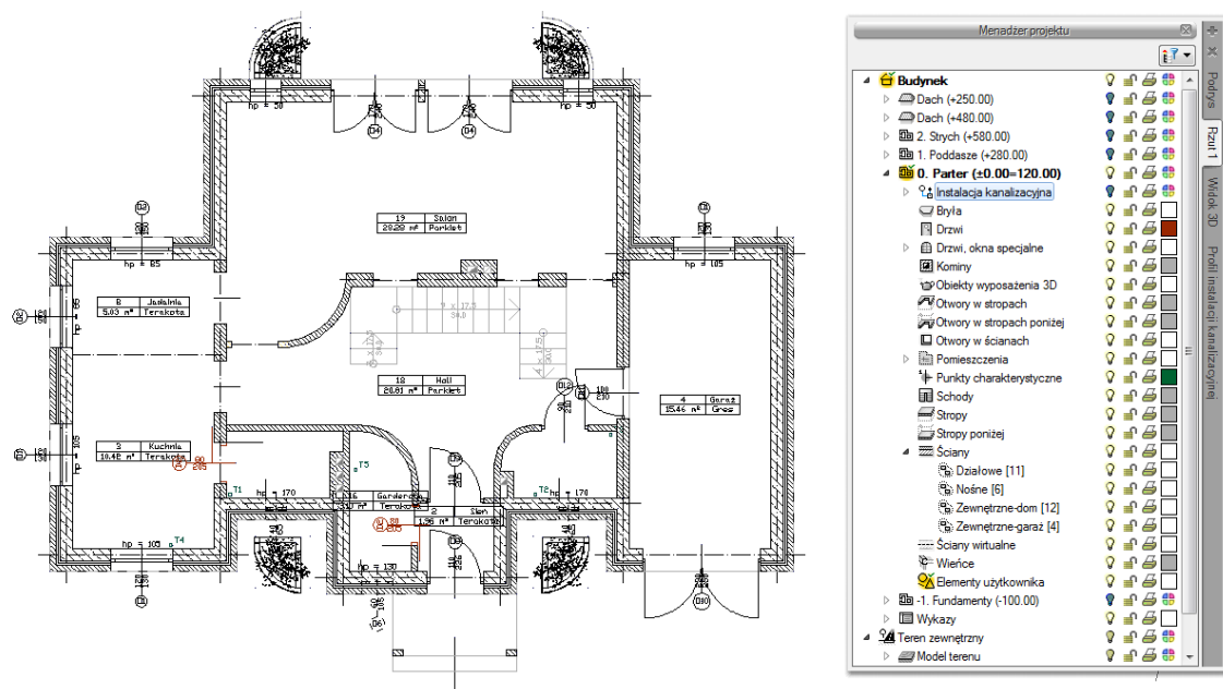
Rys. 33 Rzut kondygnacji z wyłączonymi obiektami Instalacji kanalizacyjnych
