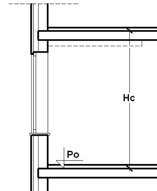
Rys. 141 Schemat danych kondygnacji, gdzie Hc jest wysokością całkowitą kondygnacji, a Po wysokością bazową (poziomym odniesieniem)
