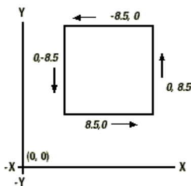
Rys. 23 Rysowanie kwadratu przy użyciu metody współrzędnych kartezjańskich względnych
