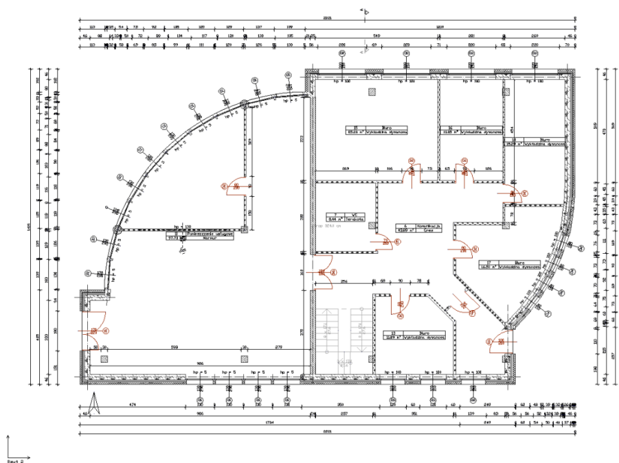
Rys. 39 Rzut kondygnacji Parter
