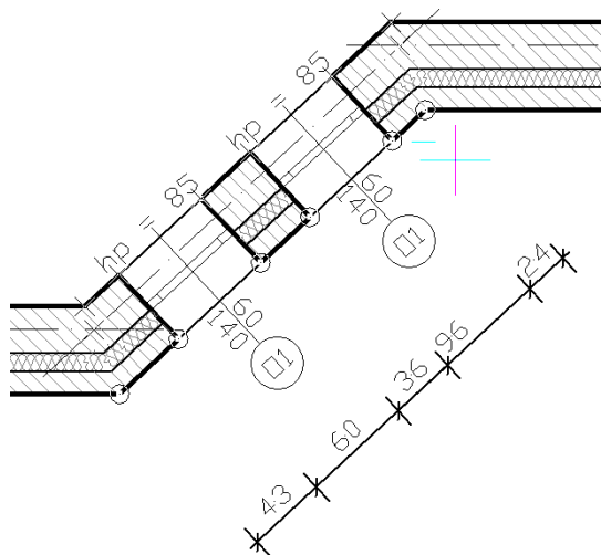
Rys. 218 Modyfikacje wymiaru
