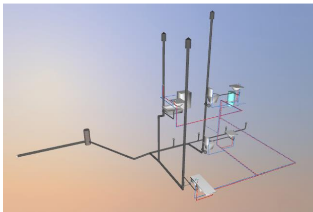
Rys. 94 Instalacja wod.-kan. w widoku z powierzchniami zdefiniowanymi w elementach
