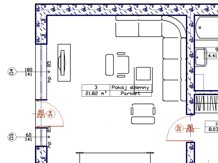
Rys. 204 Przykład rzutu kondygnacji z włączonym wyświetlaniem grubości linii
