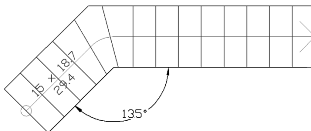
Rys. 223 Zwymiarowany element
