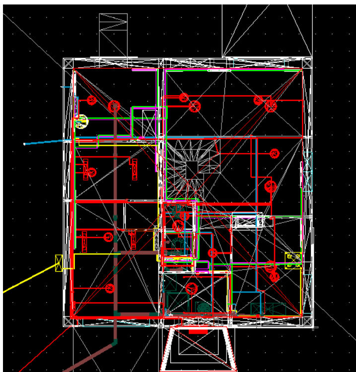
Rys. 255 Widok rzutu modelu IFC z widocznymi wszystkimi krawędziami
