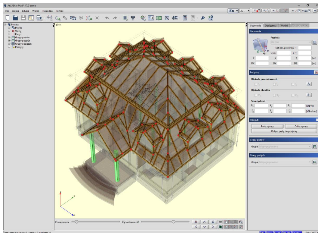
Rys. 276 Przykładowy projekt po przejściu do programu R3D3-Rama 3D
