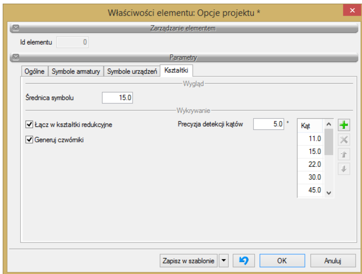
Rys. 87. Okno Opcje projektu, zakładka Kształtki
