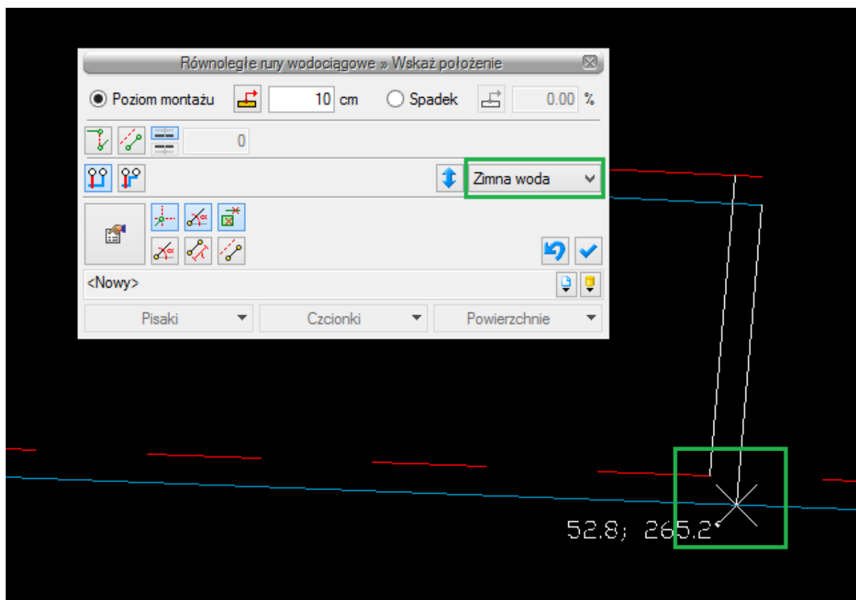
Rys. 81. Rysunek przedstawiający wstawianie równoległych rur wodociągowych z wiodącym rurociągiem wody zimnej
