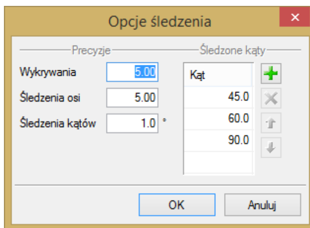
Rys. 5. Okno opcji śledzenia
