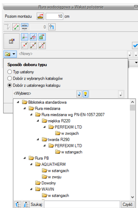
Rys. 94. Okno przełączania sposobu doboru parametrów, sposób wyboru Dobór z ustalonego katalogu
