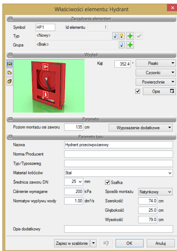
Rys. 54. Okno właściwości elementu Hydrant
