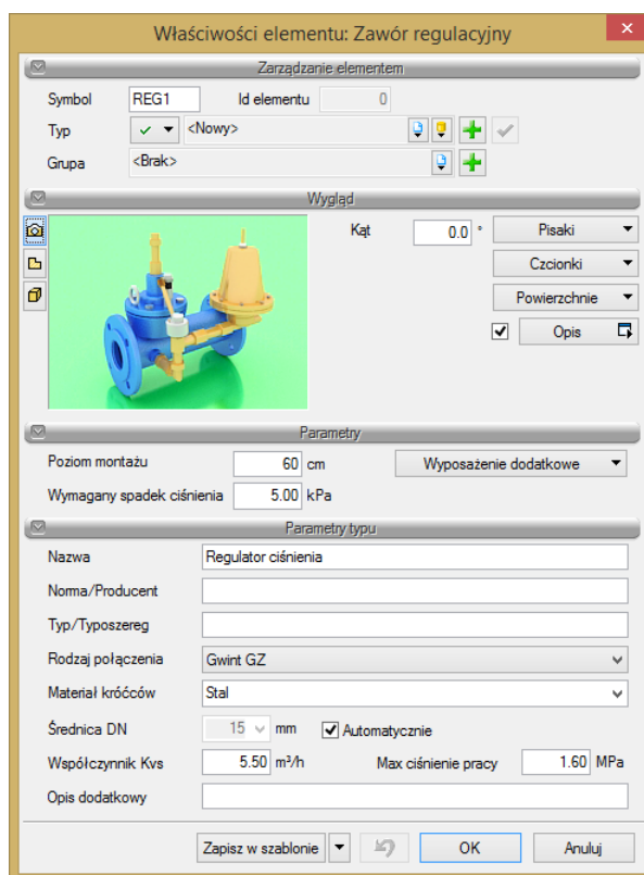
Rys. 61. Okno właściwości elementu Zawór regulacyjny
