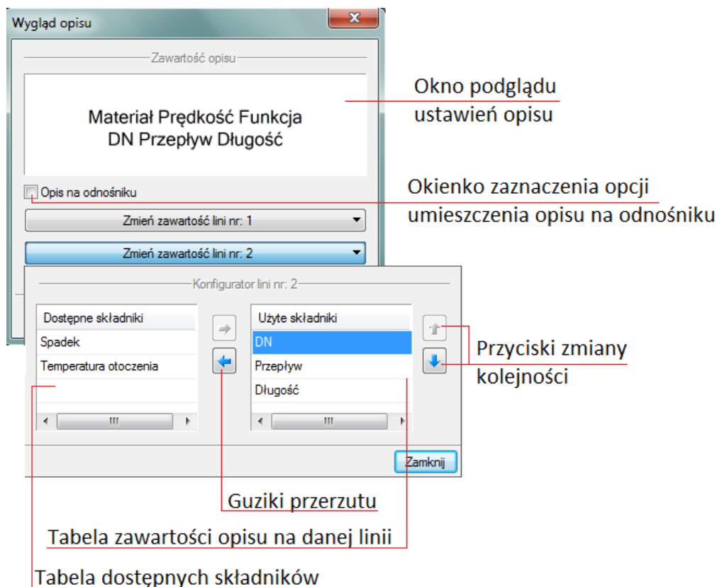
Rys. 32. Konfigurator opisów, widok okna ustawienia
