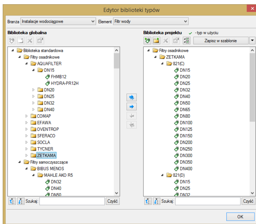
Rys. 12. Okno Edytora biblioteki typów
