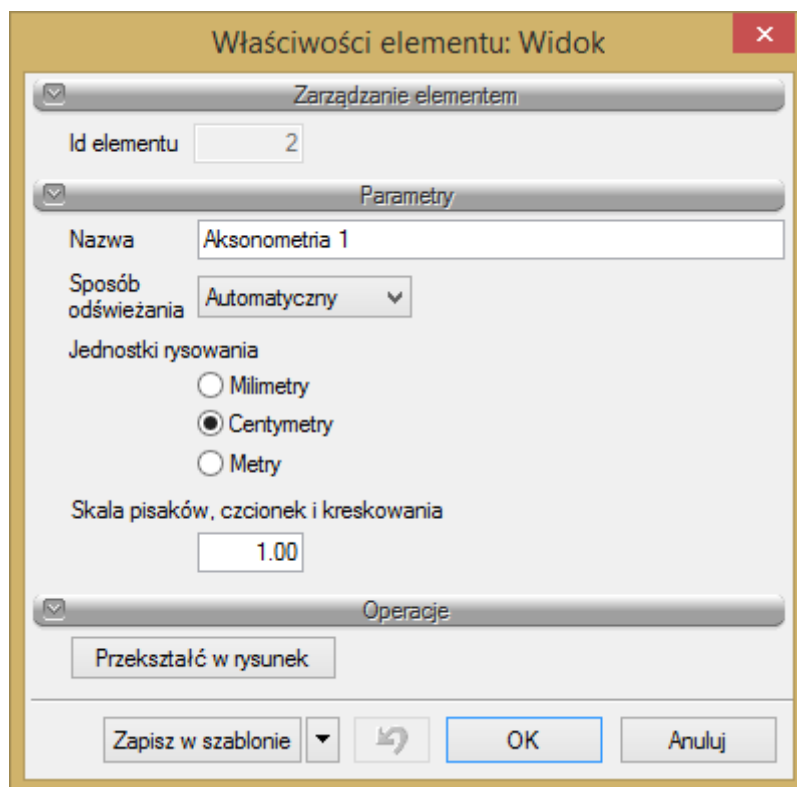
Rys. 116. Okno właściwości widoku aksonometrii
