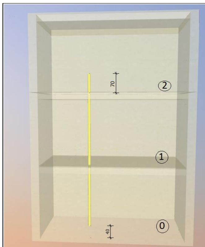
Rys. 42. Widok 3D pionu rozciągniętego na inne kondygnacje za pomocą funkcji Rozciągnij pion
