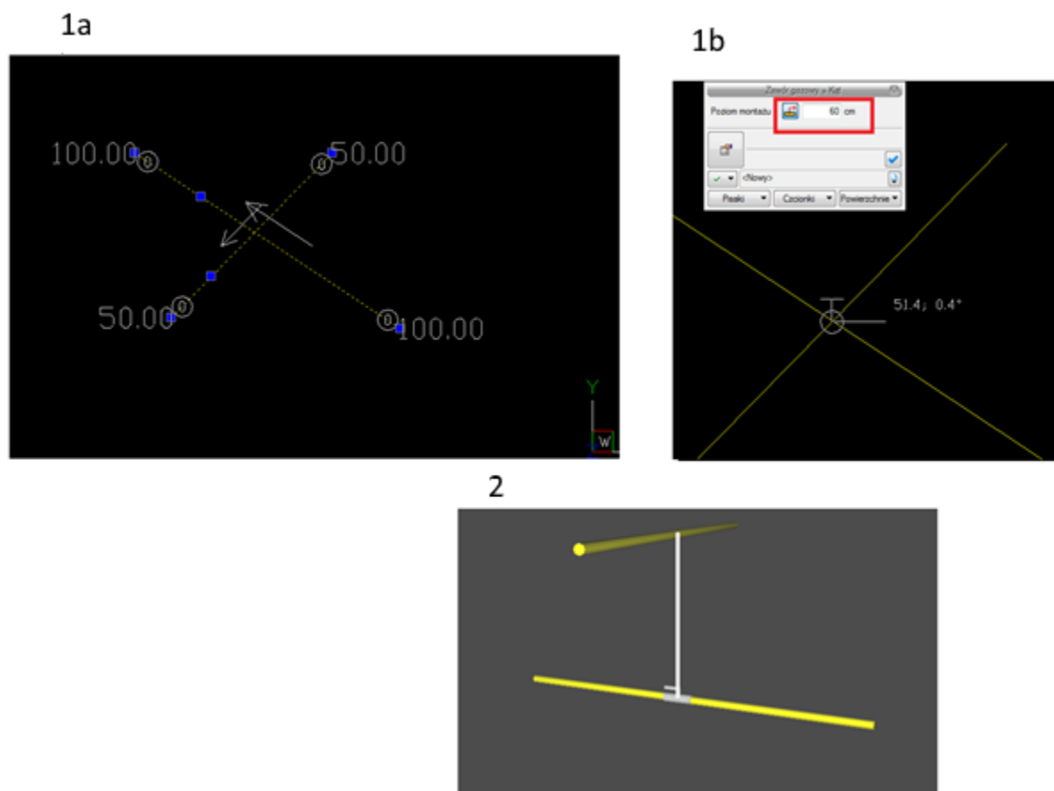
Rys. 12. Przykład zastosowania funkcji Pobierz z elementu podczas wstawiania zaworu na jeden z krzyżujących się w planie rurociągów poziomych. 1a – Widok w polu rysunkowym dwóch rurociągów krzyżujących się na poziomach 50 cm i 100 cm, 1a – Schemat wstawienia zaworu na rurociąg z poziomu 50 cm., 2 – Rezultat wstawienia zaworu na 3D.
