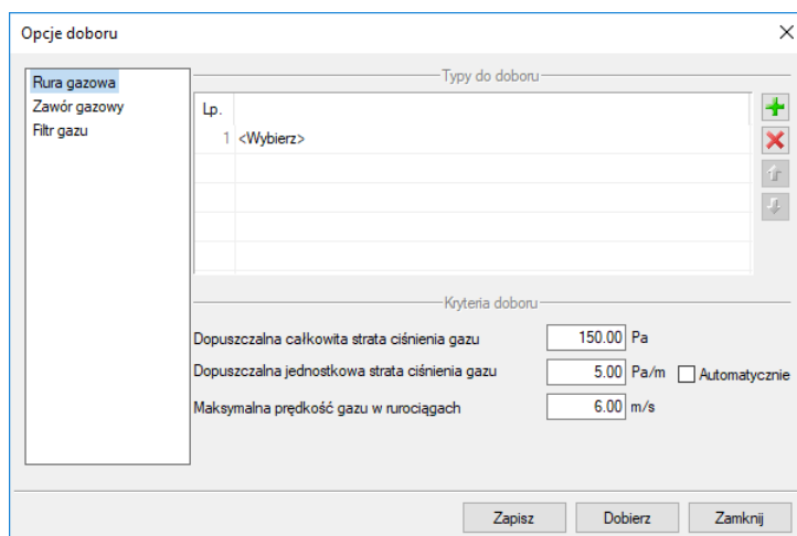
Rys. 55. Okno opcji doborów, ustawianie kryteriów doboru
