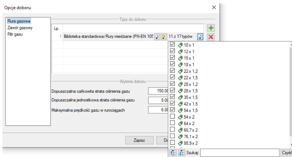
Rys. 56. Okno opcji doboru, wybór typów elementu do doboru
