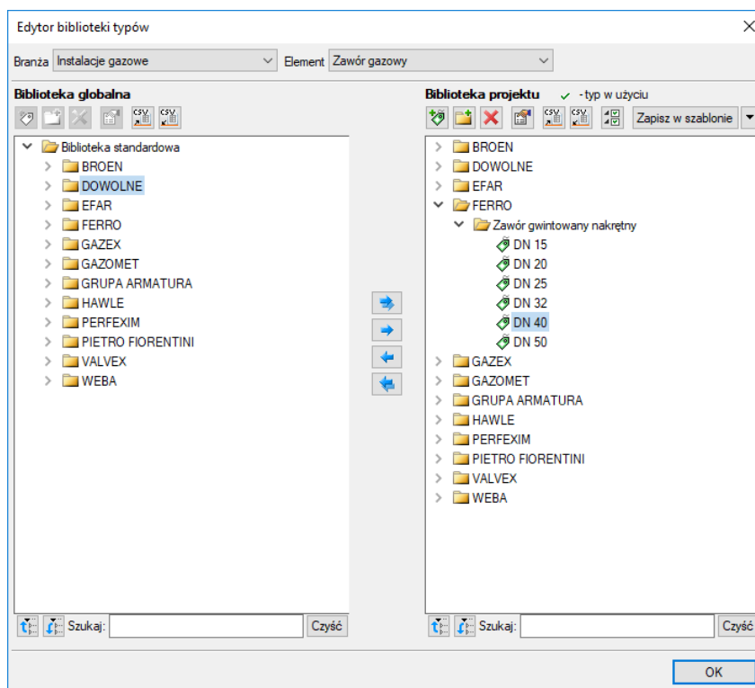
Rys. 46. Okno edytora biblioteki typów po wybraniu odpowiedniej branży i jednego z jej elementów
